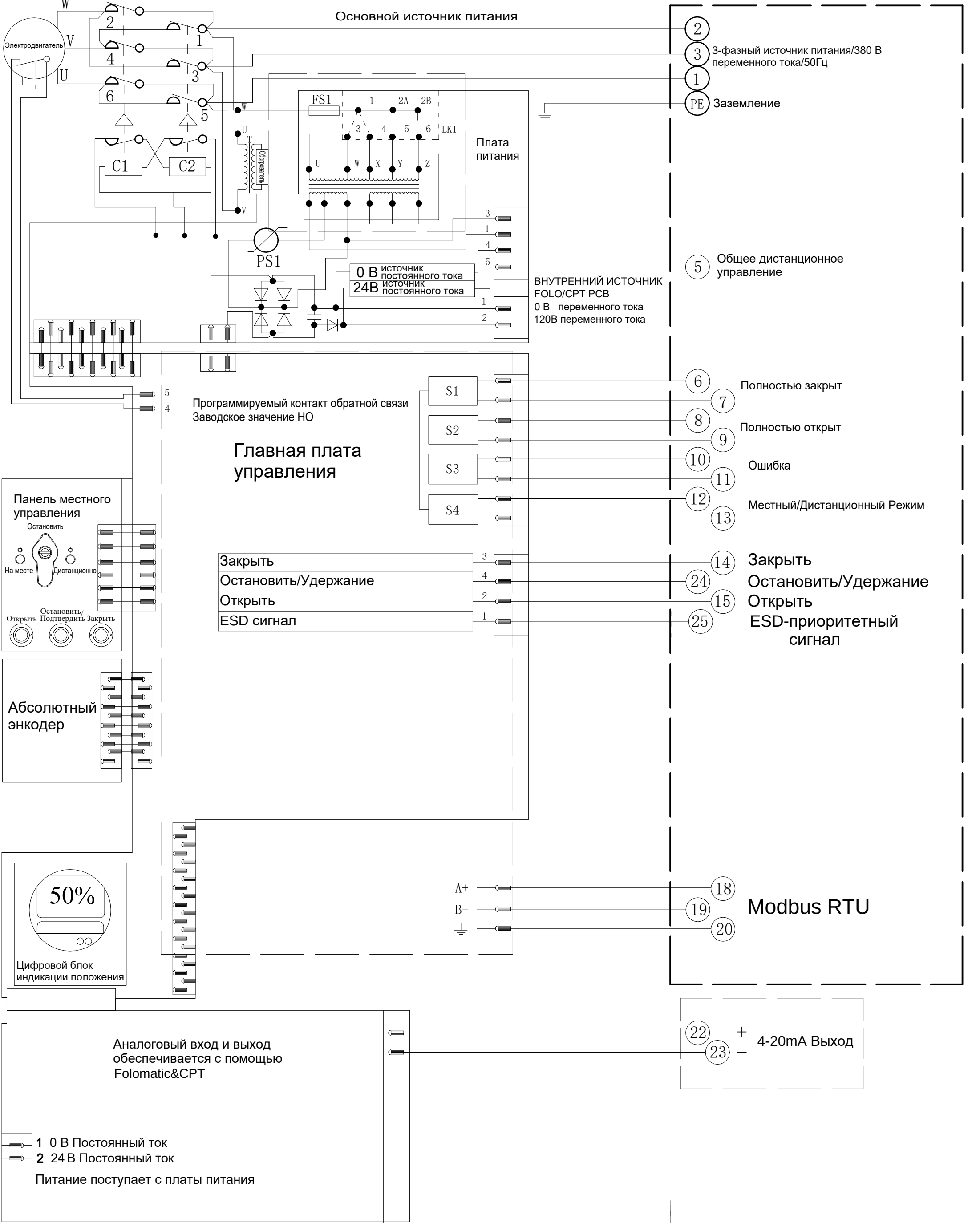
Электрическая схема №8-380-24-4-MR-3 Серия VADQM006-030/100-200
