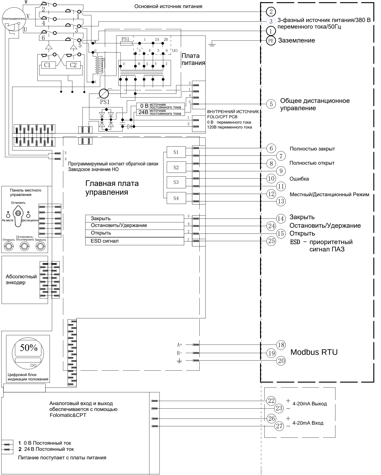
Электрическая схема №8-380-24-4-MR-1 Серия VADQM006-030/100-200
