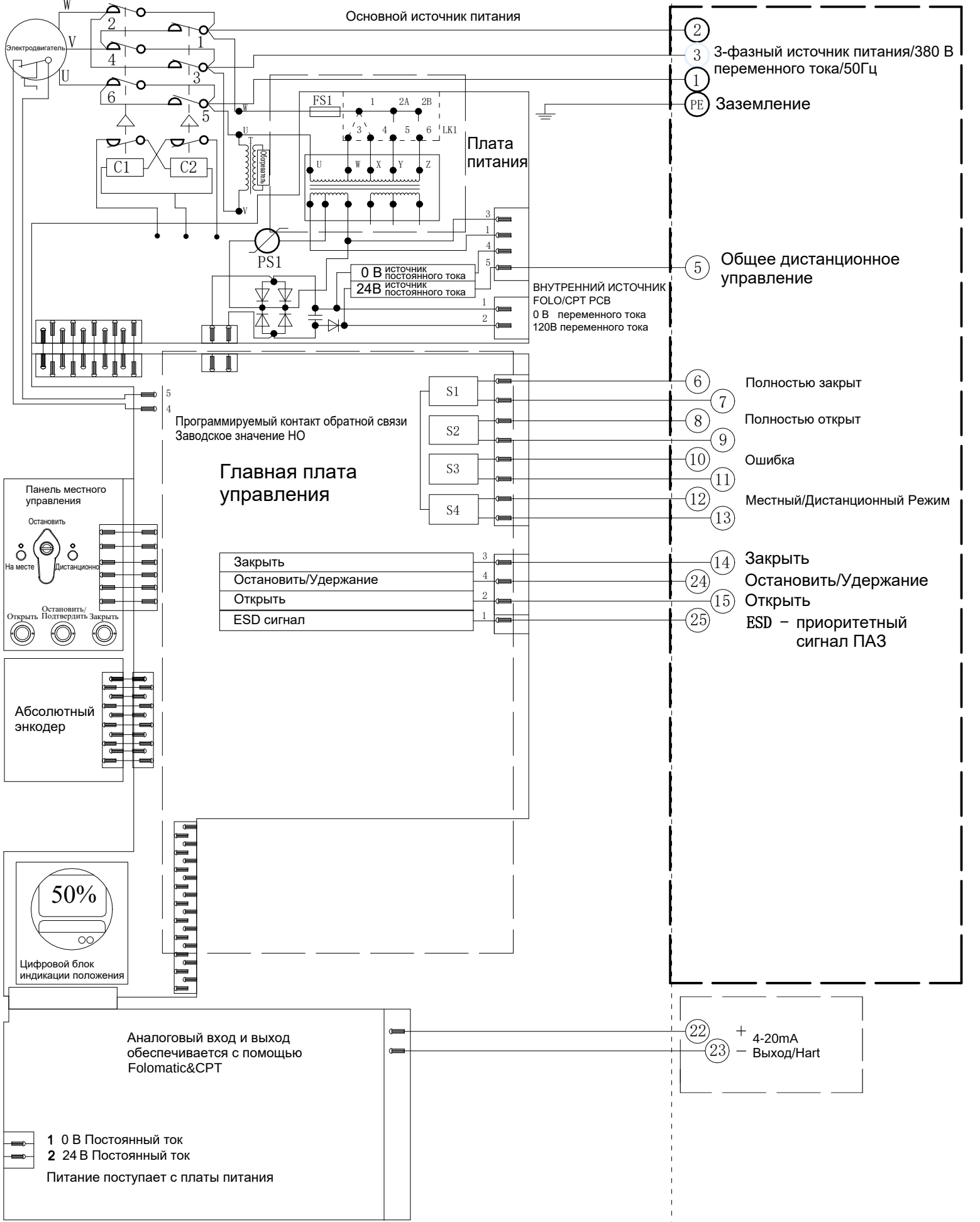
Электрическая схема №8-380-24-4-HR-3 Серия VADQM006-030/100-200
