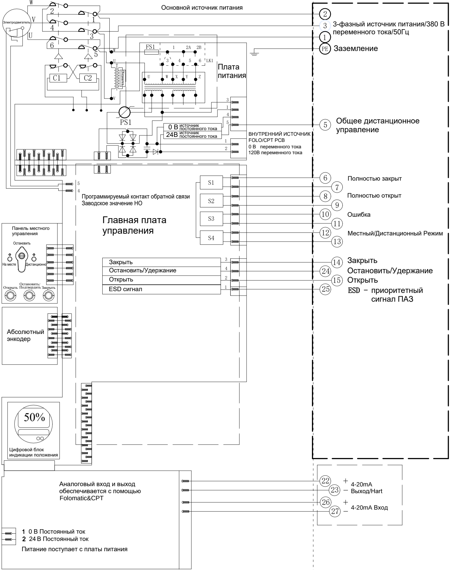
Электрическая схема №2-380-24-4-HR-1 Серия VADQM006-030/100-200
