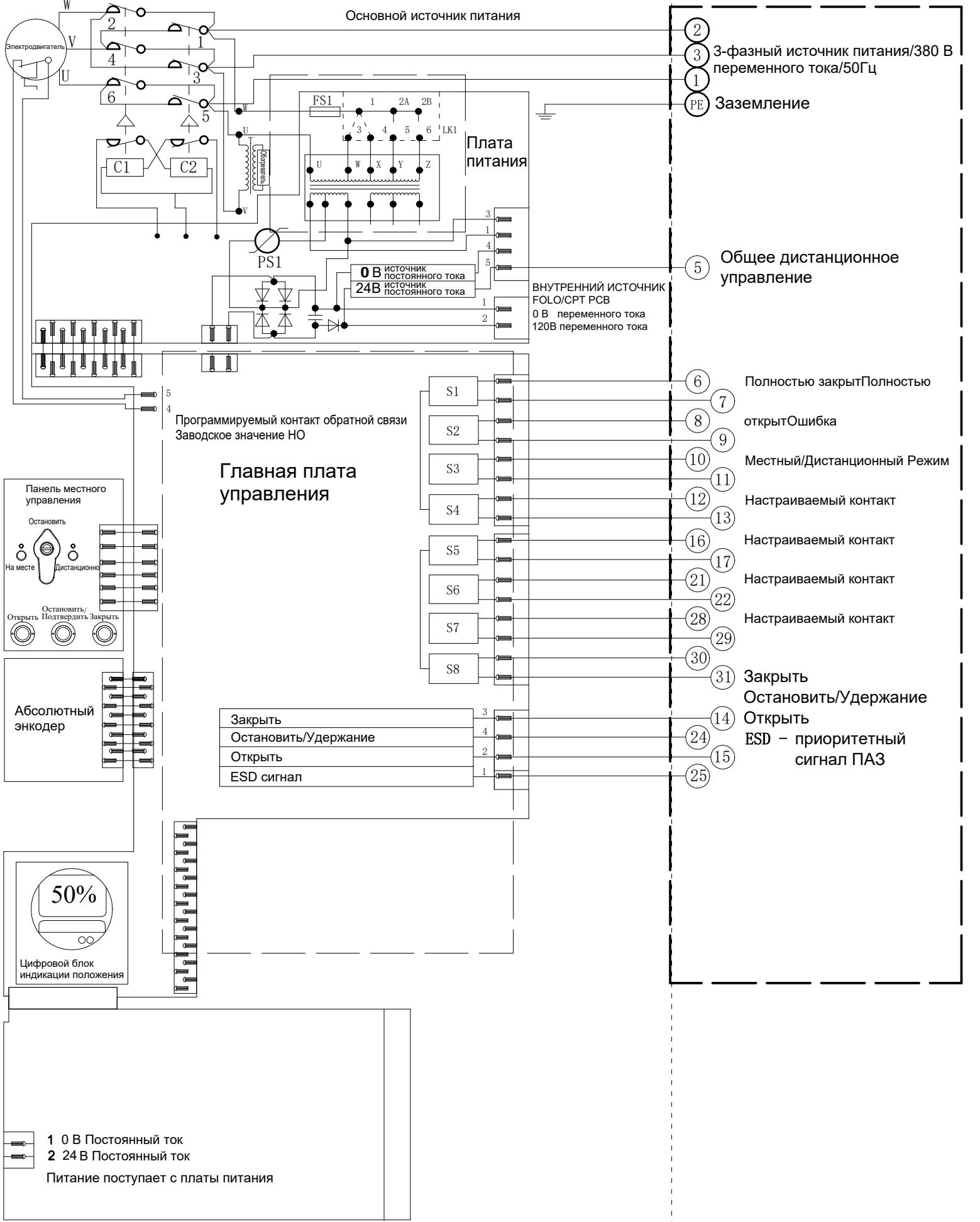
Электрическая схема №8-380-24-8-N-0 Серия VADQM006-030/100-200
