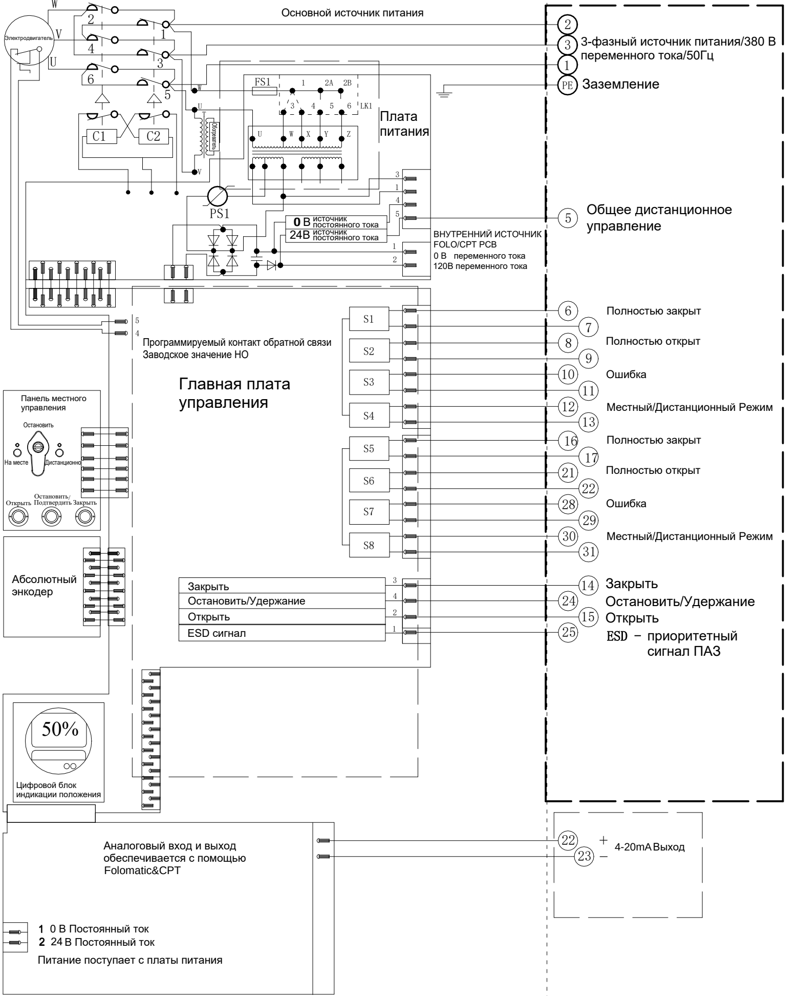
Электрическая схема №8-380-24-8-N-3 Серия VADQM006-030/100-200
