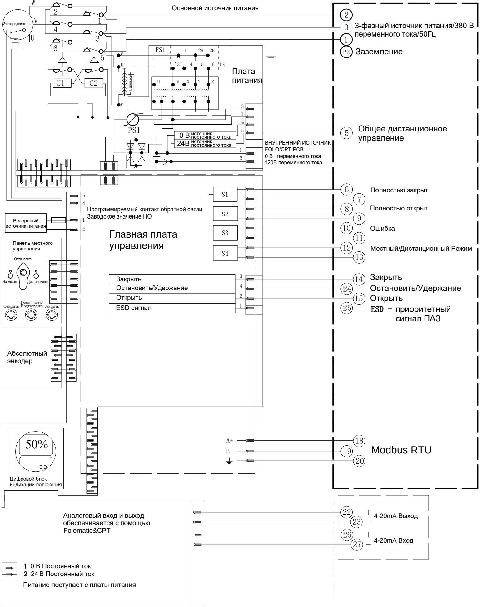
Электрическая схема №8-380В-24-4-MR-1 Серия VADQM006-030/100-200
