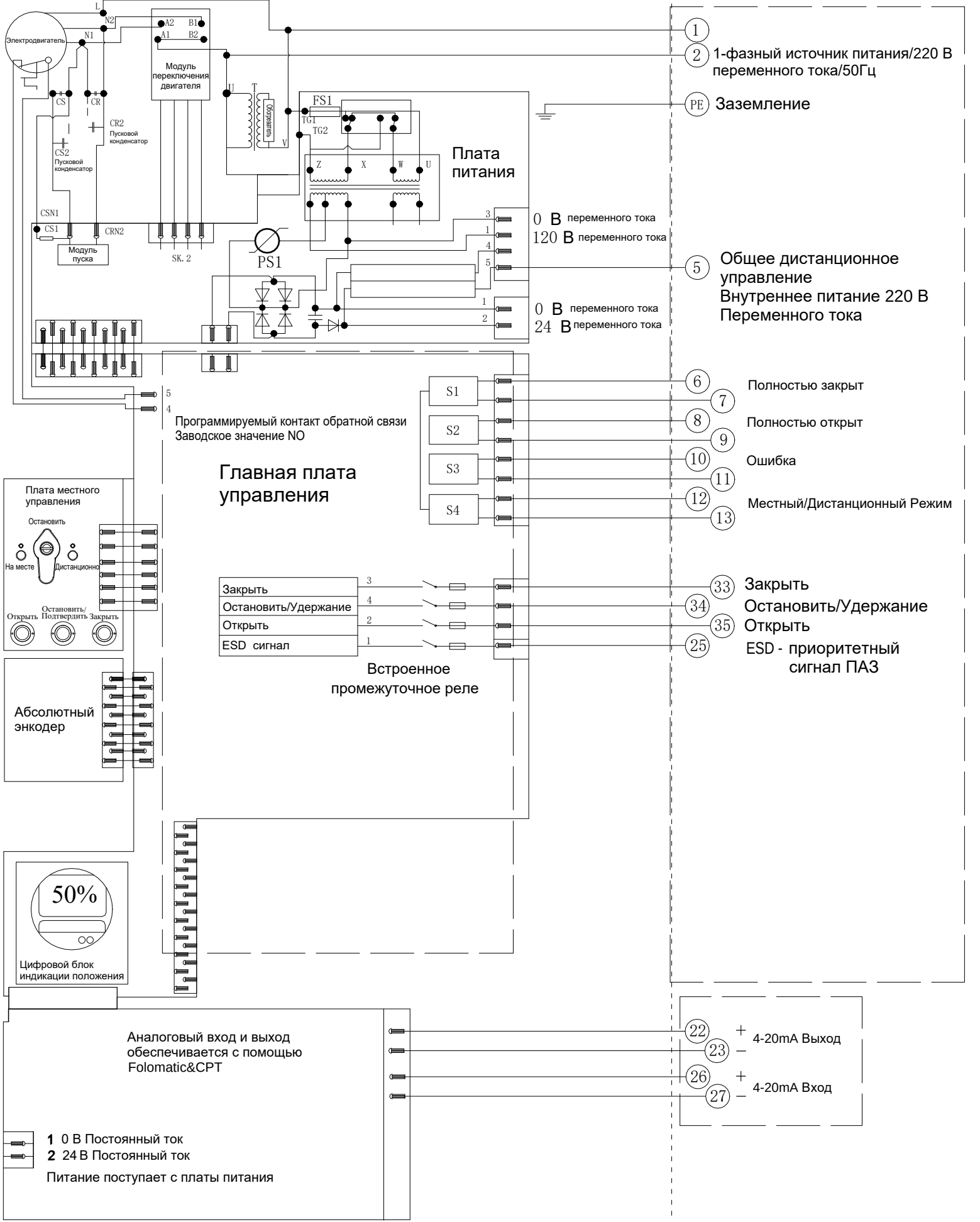
Электрическая схема №8-220-220-4-N-1 Серия VADQM006-030/100-200
