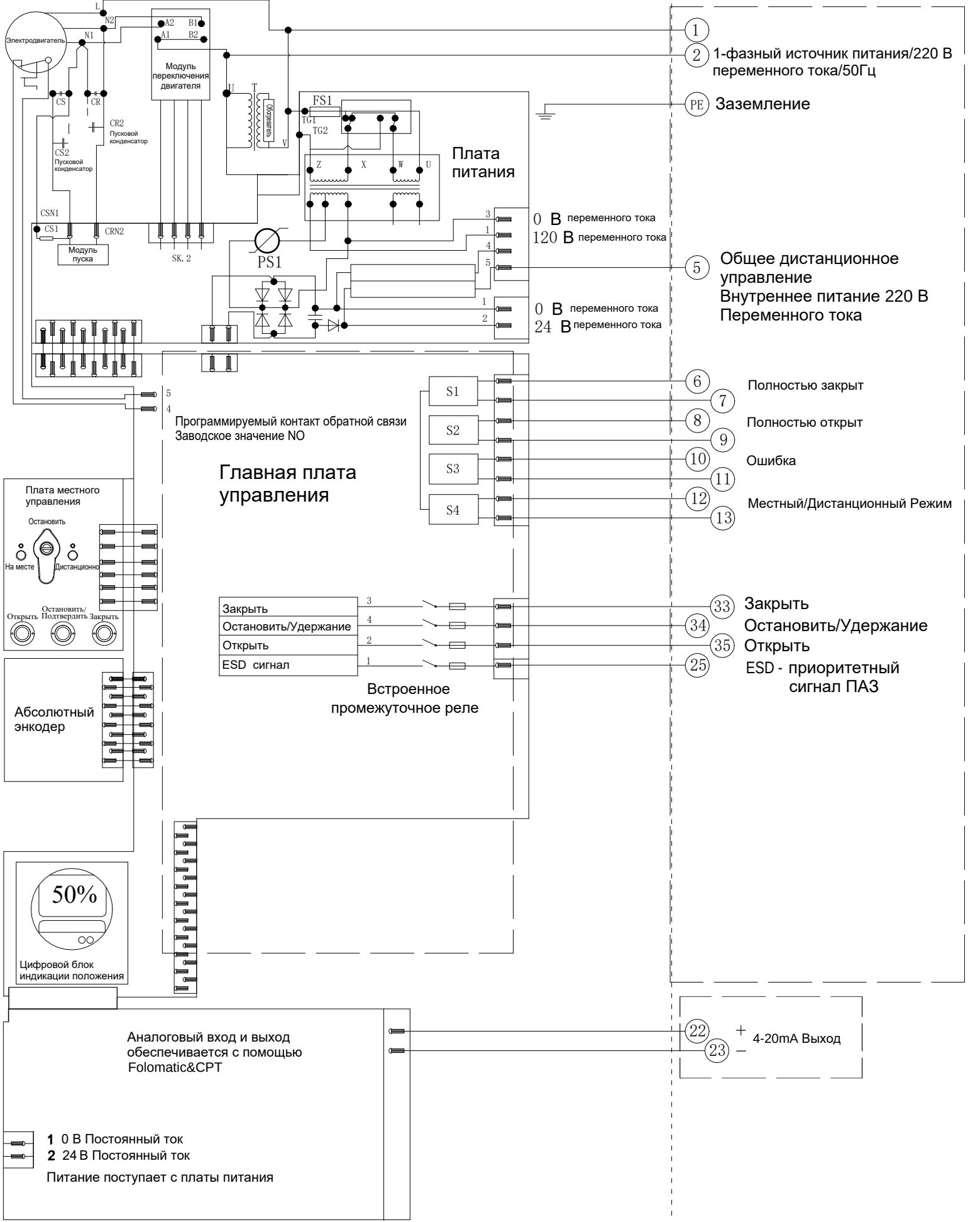
Электрическая схема №8-220-220-4-N-3 Серия VADQM006-030/100-200
