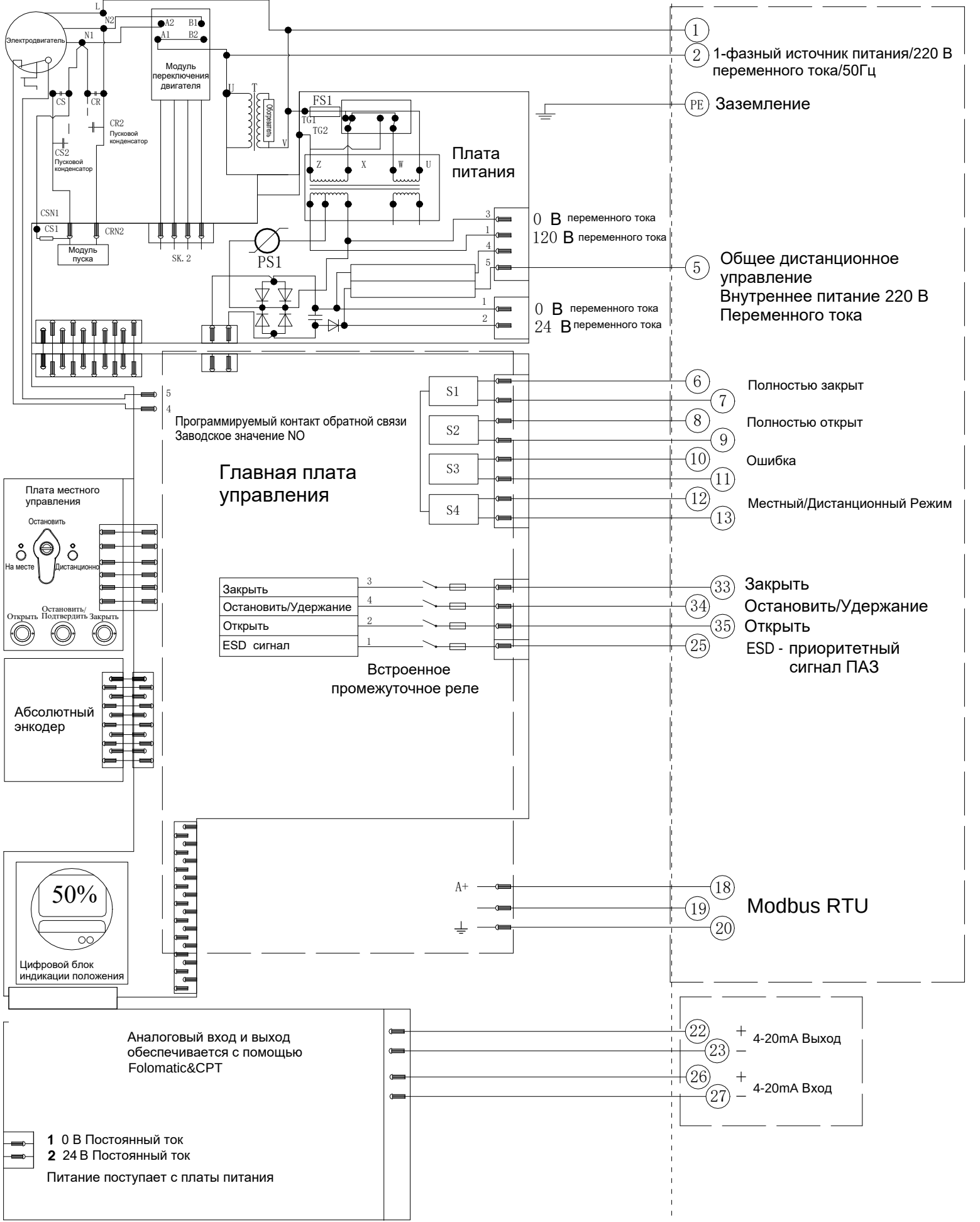
Электрическая схема №8-220-220-4-MR- 1 Серия VADQM006-030/100-200
