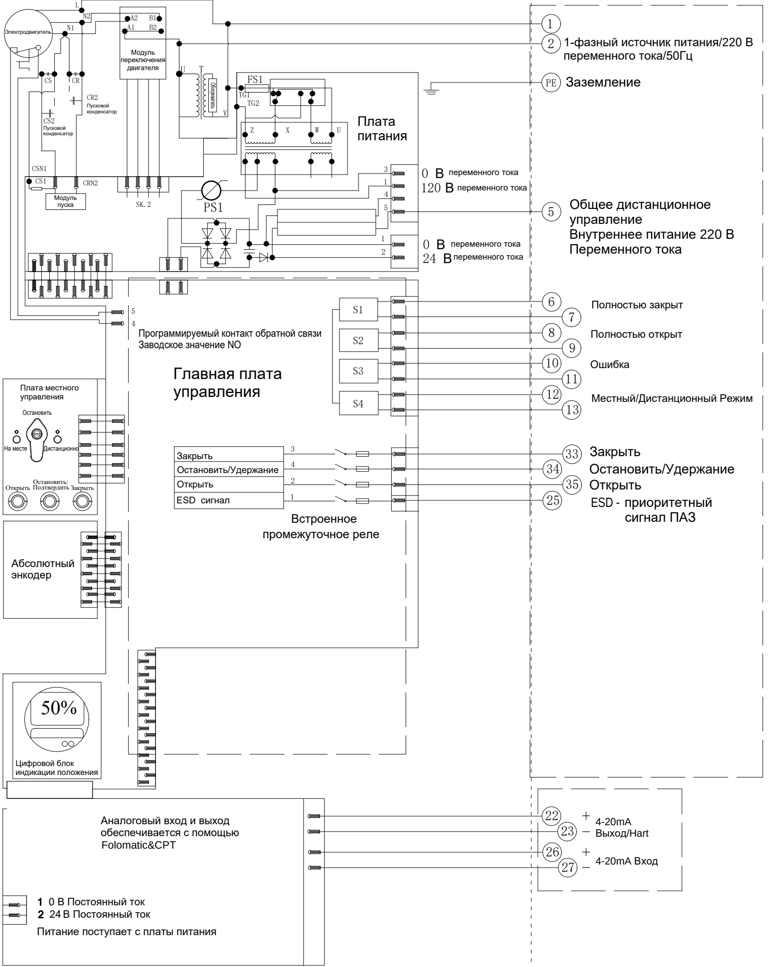
Электрическая схема №8-220-220-4-HR- 1 Серия VADQM006-030-100-200
