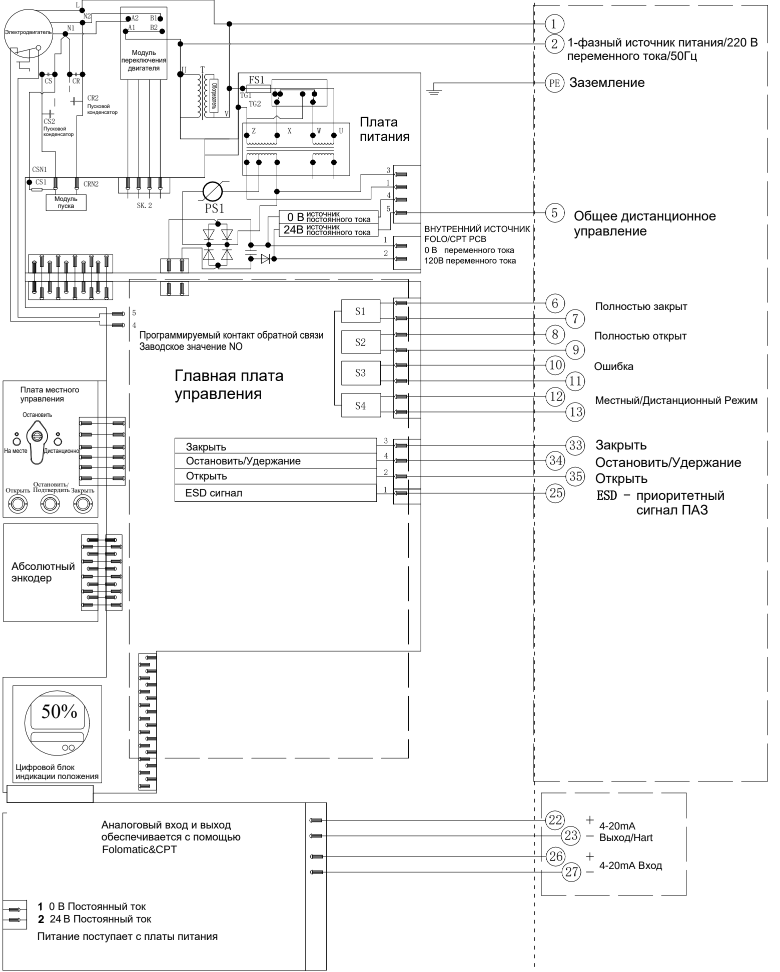
Электрическая схема №8-220-24-4-HR-1 Серия VADQM006-030-100-200
