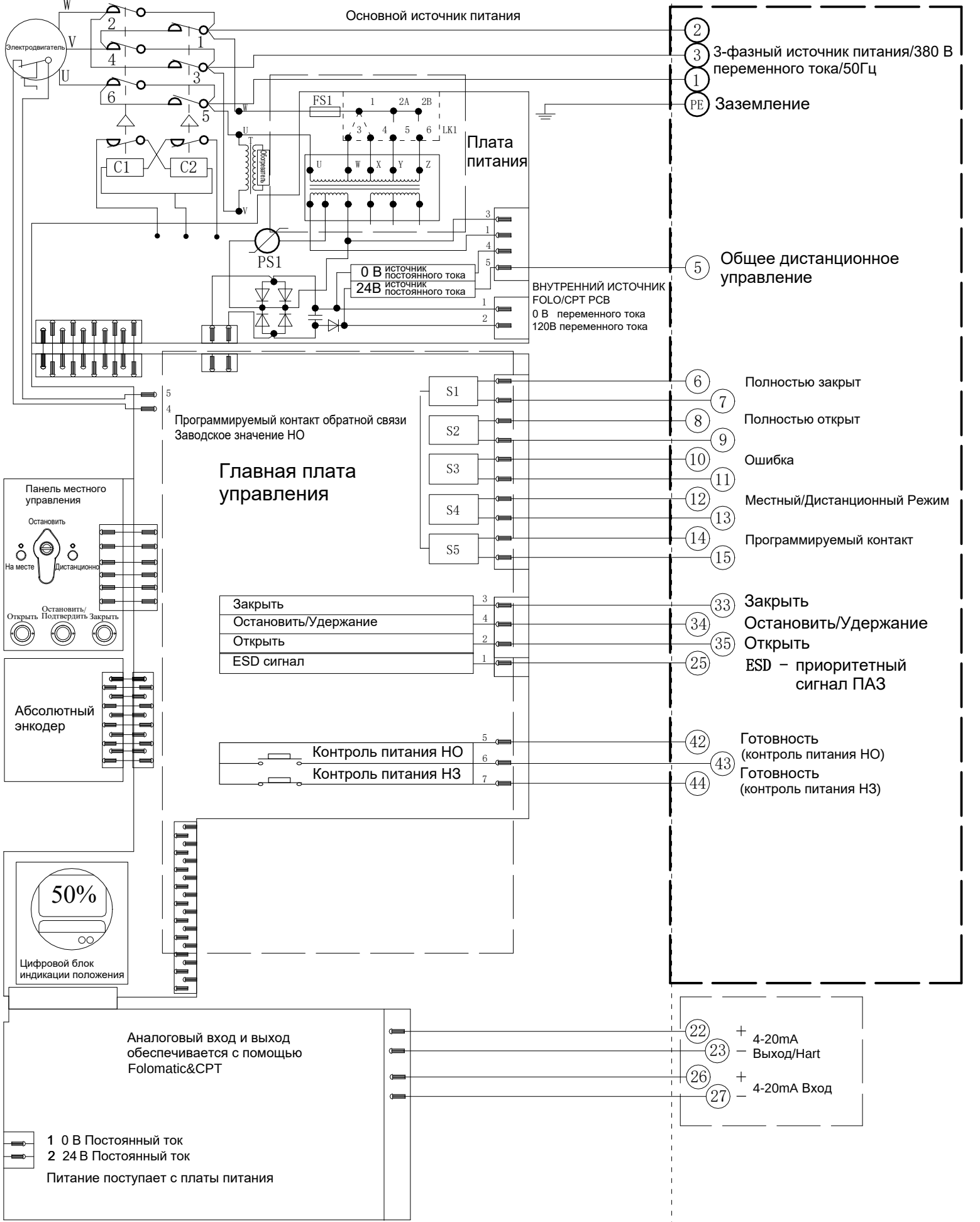
Электрическая схема №9-380-24-6-HR-1 Серия VADQM040/060/080
