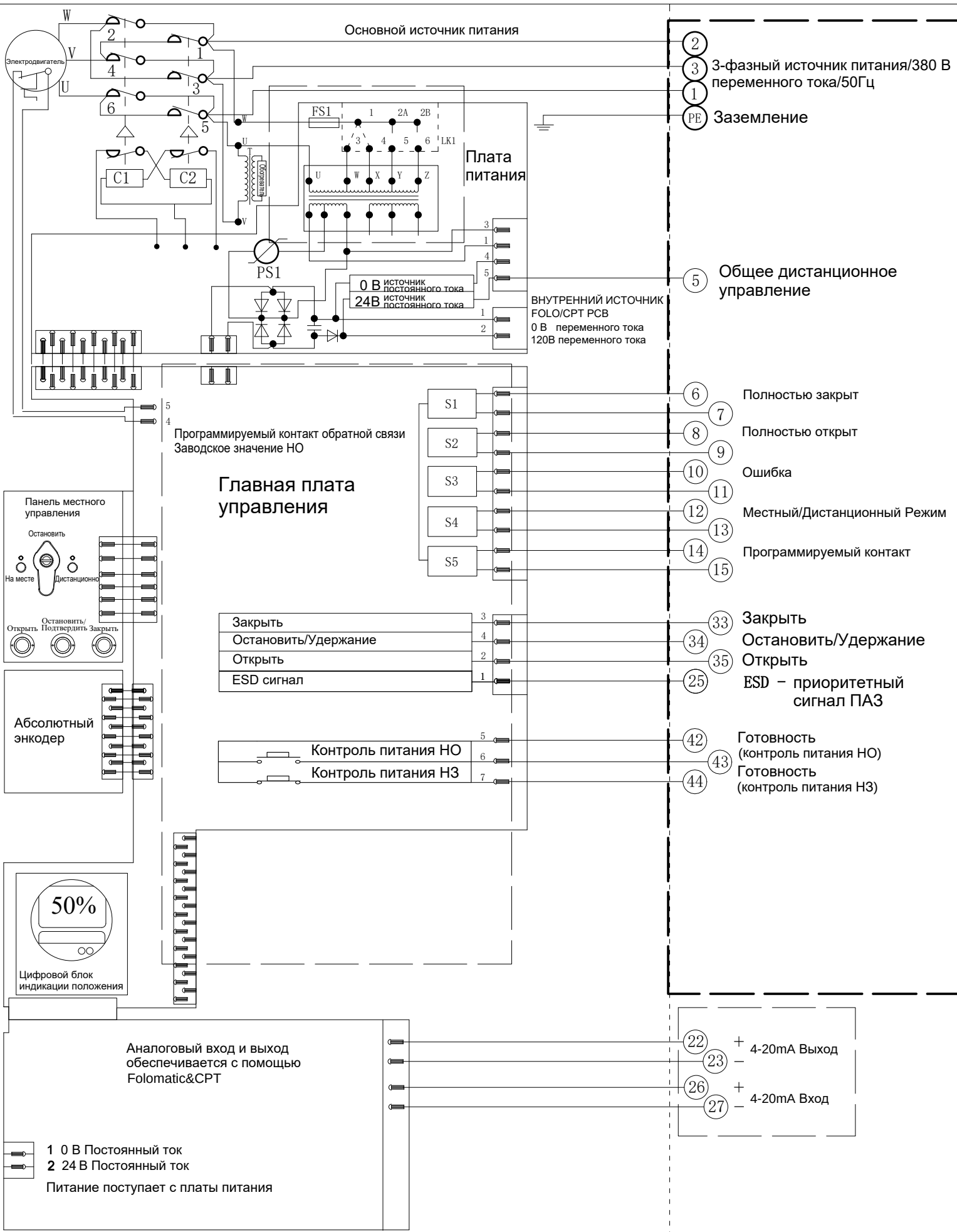
Электрическая схема №9-380-24-6-N-1 Серия VADQM040/060/080
