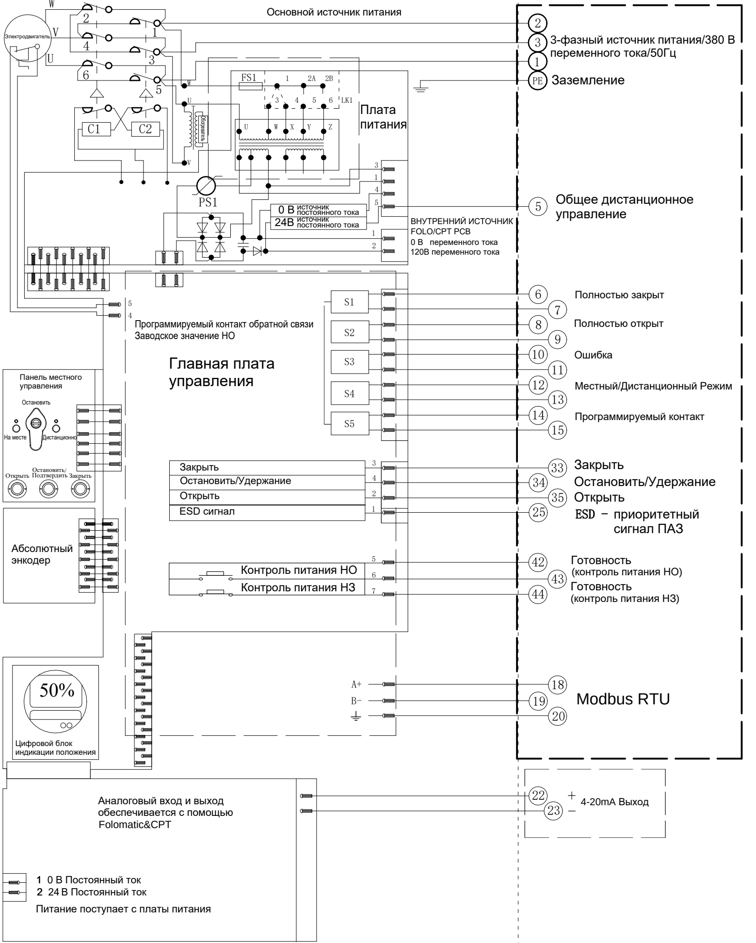
Электрическая схема №9-380-24-6-MR-3 Серия VADQM040/060/080
