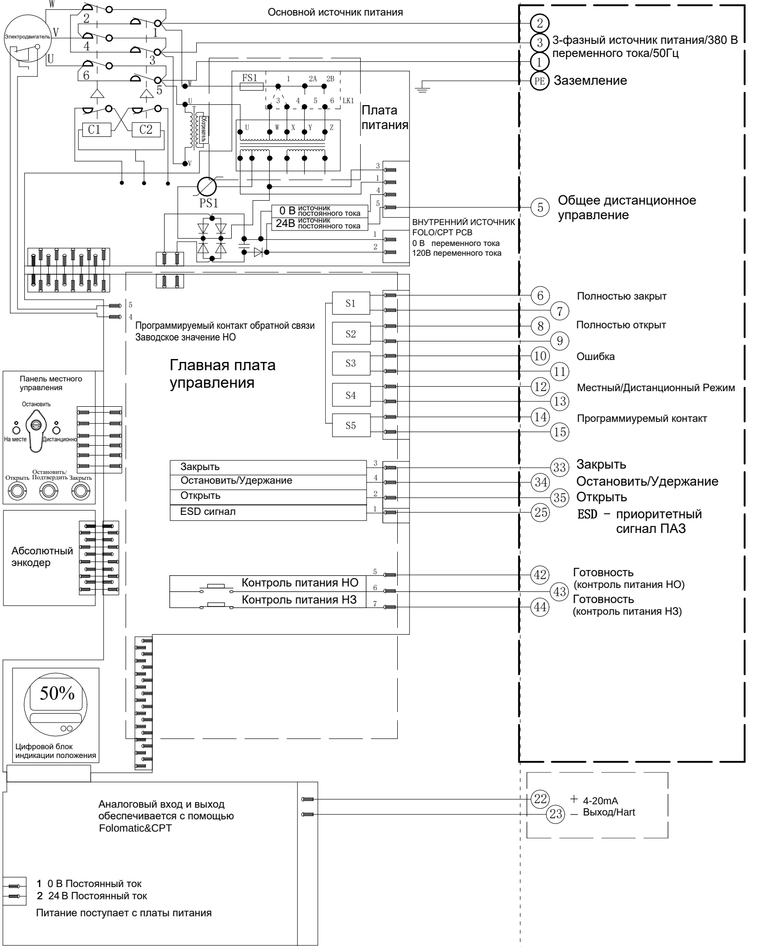
Электрическая схема №9-380-24-6-HR-3 Серия VADQM040/060/080
