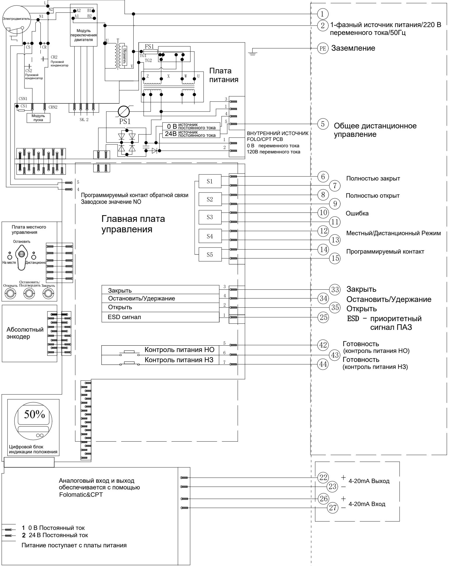
Электрическая схема №9-220-24-6-N-1 Серия VADQM040/060/080
