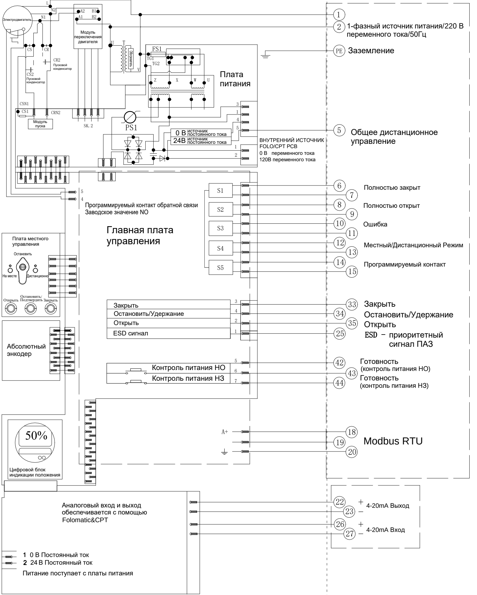
Электрическая схема №9-220-24-6-MR-1 Серия VADQM040/060/080
