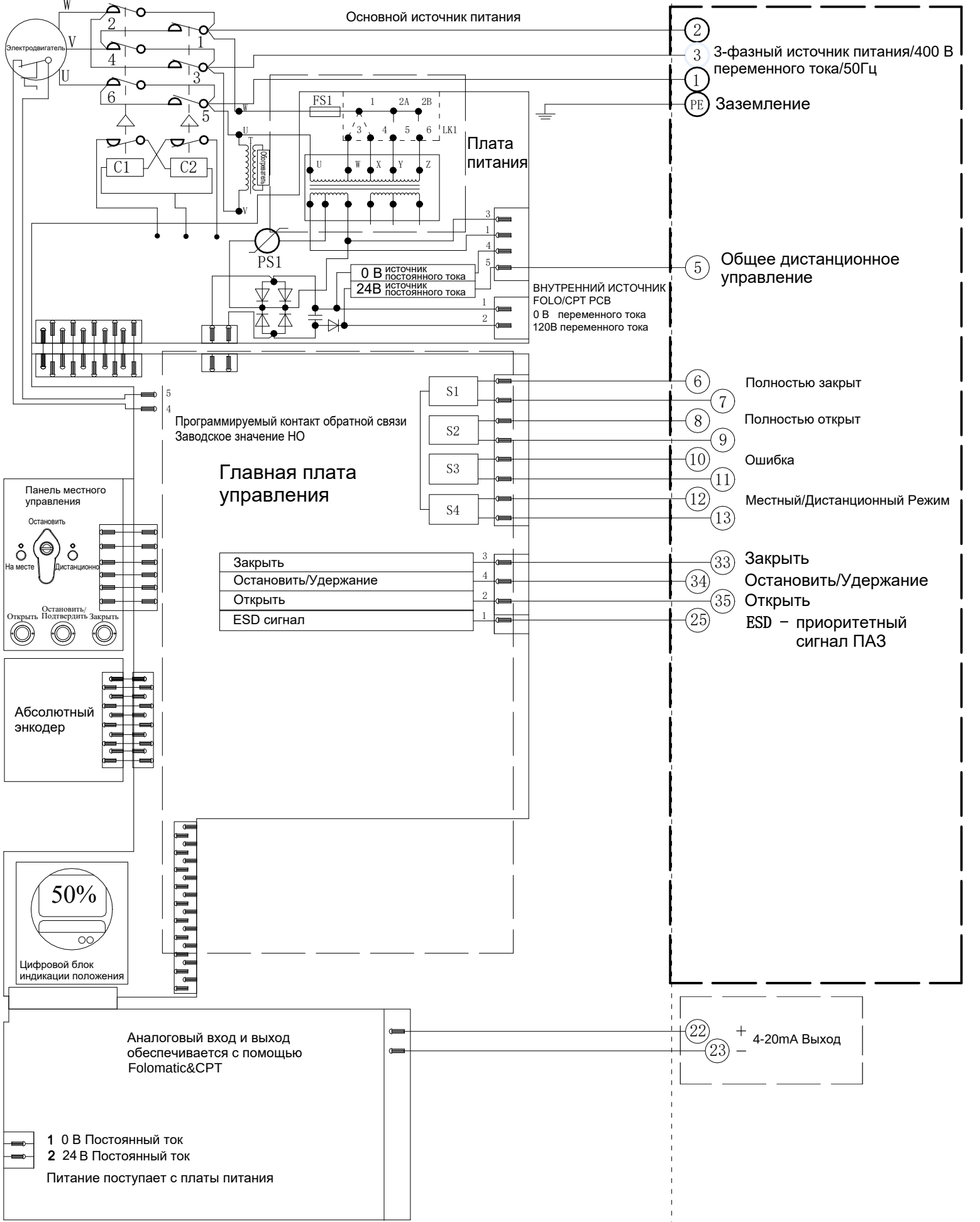
Электрическая схема №9-400-24-4-N-3 Серия VADQM040/060/080
