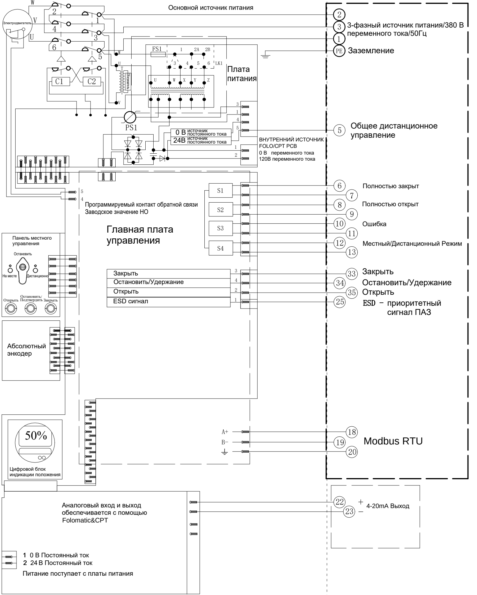
Электрическая схема №9-380-24-4-MR-3 Серия VADQM040/060/080
