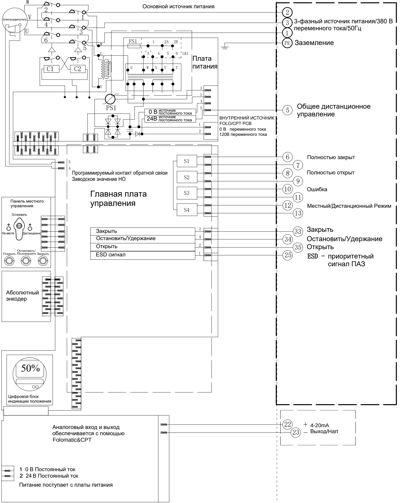
Электрическая схема №9-380-24-4-HR-3 Серия VADQM040/060/080
