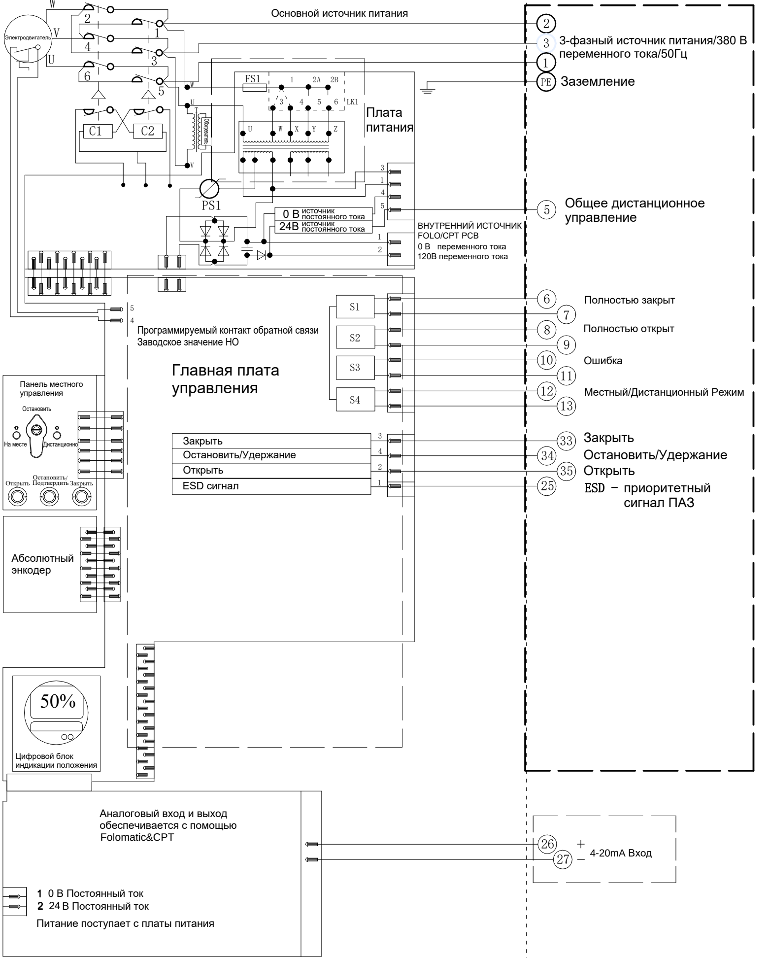
Электрическая схема №9-380-24-4-N-2 Серия VADQM040/060/080
