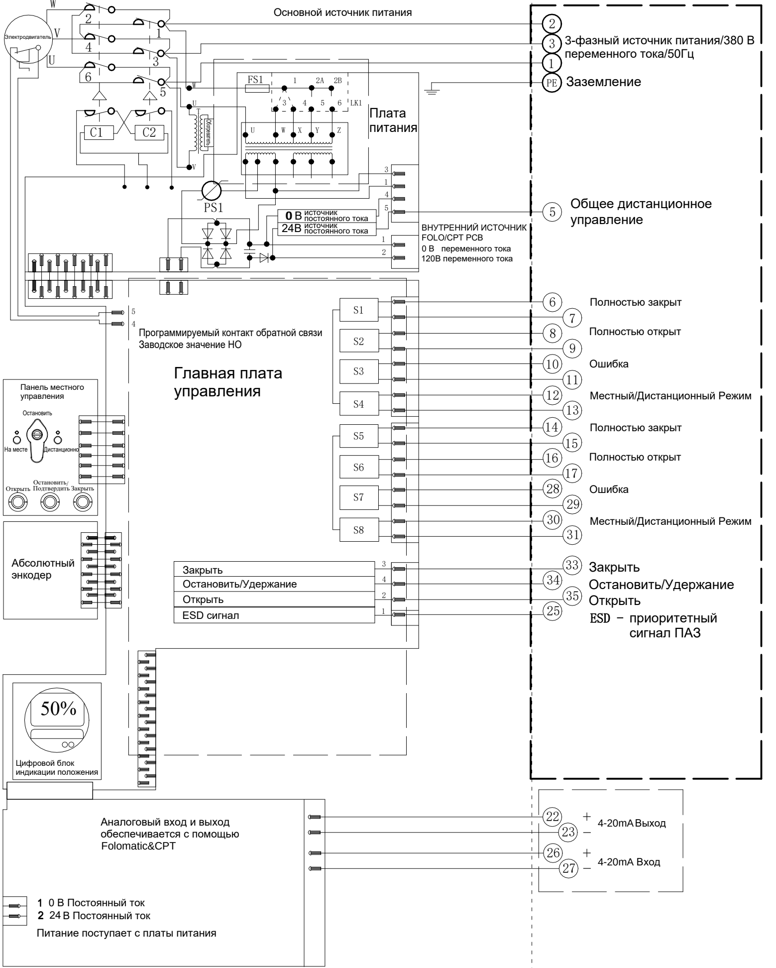
Электрическая схема №9-380-24-4-N-1 Серия VADQM040-080
