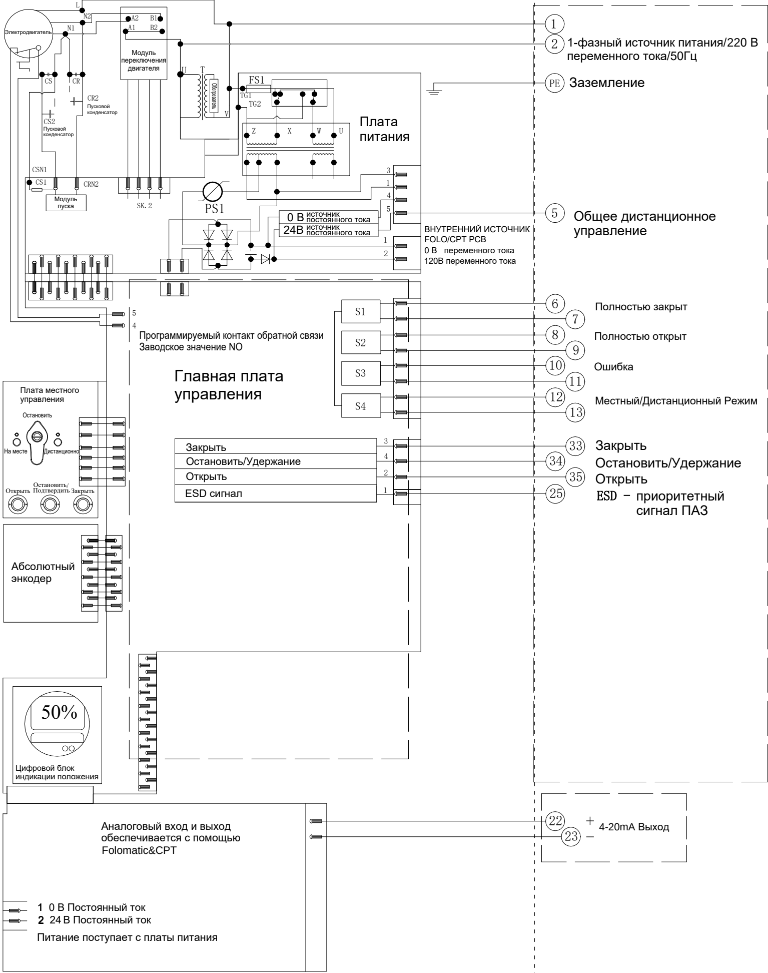
Электрическая схема №9-220-24-4-N-3 Серия VADQM040/060/080
