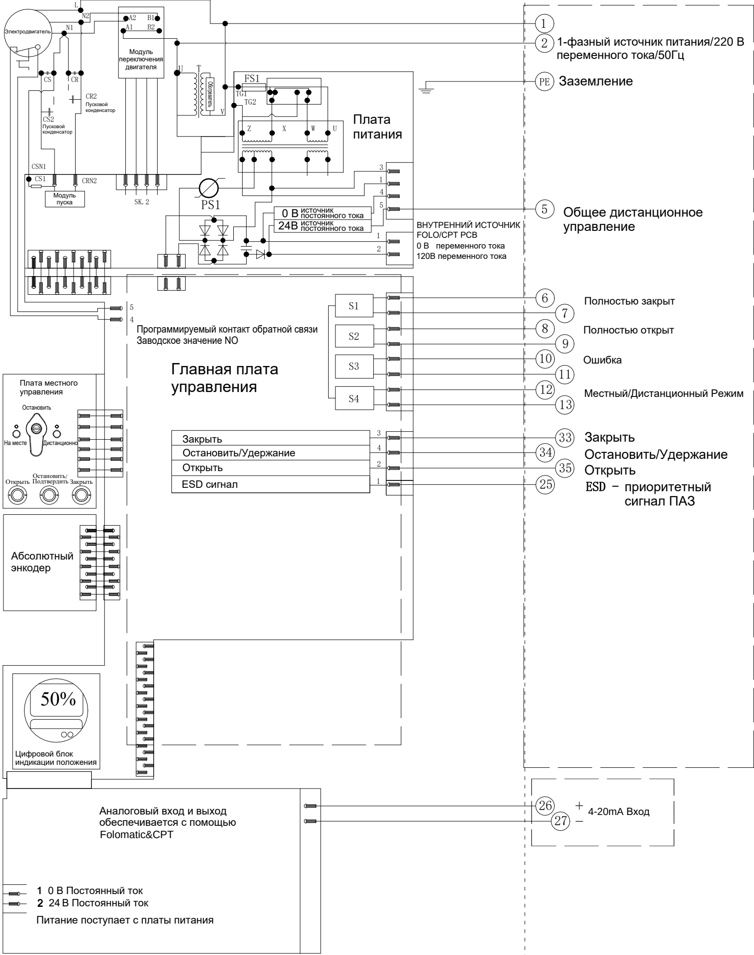
Электрическая схема №9-220-24-4-N-2 Серия VADQM040/060/080
