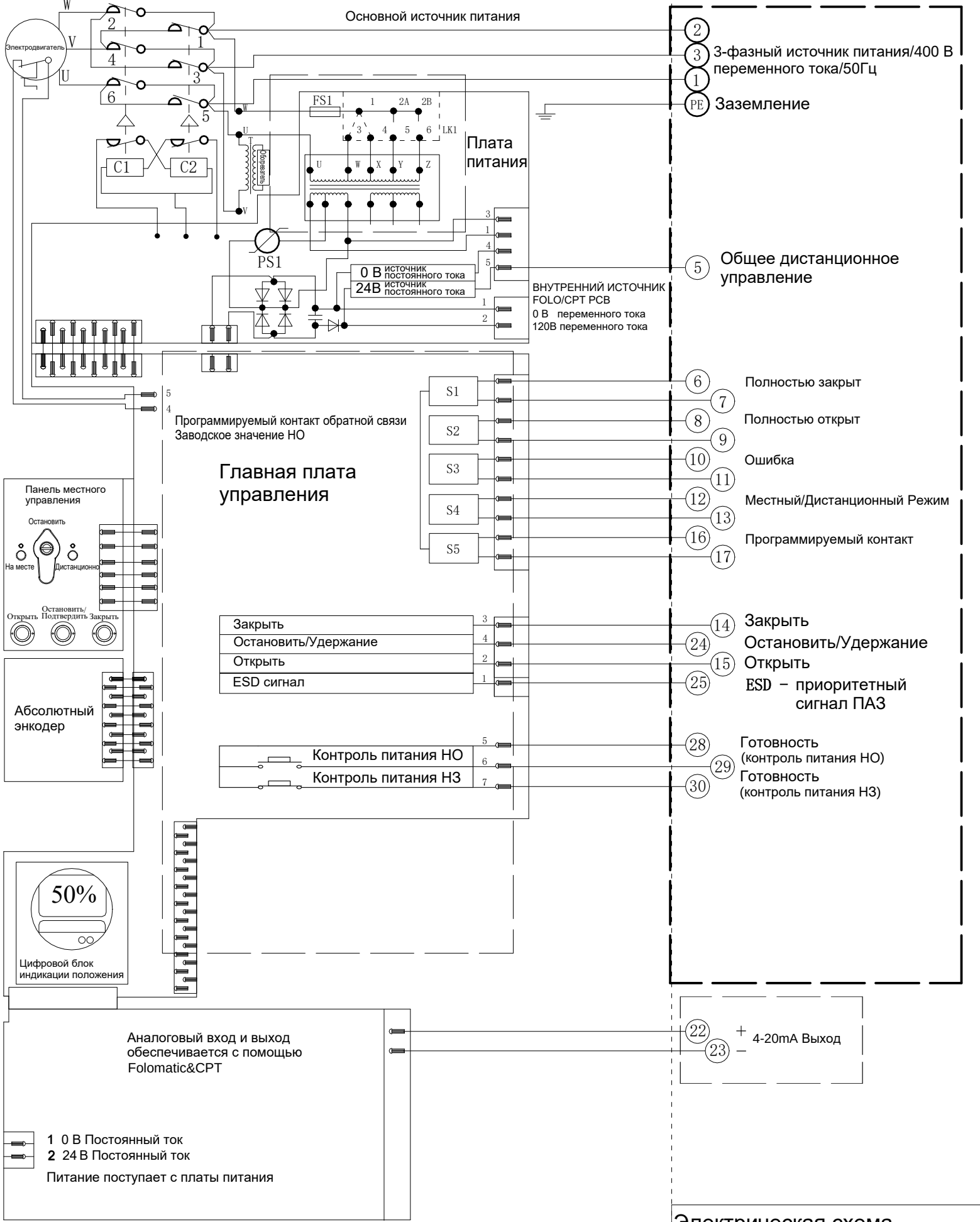
Электрическая схема №2-400-24-6-N-3 Серия VADQ006-010-015-020-030/ VADQ100-150-200
