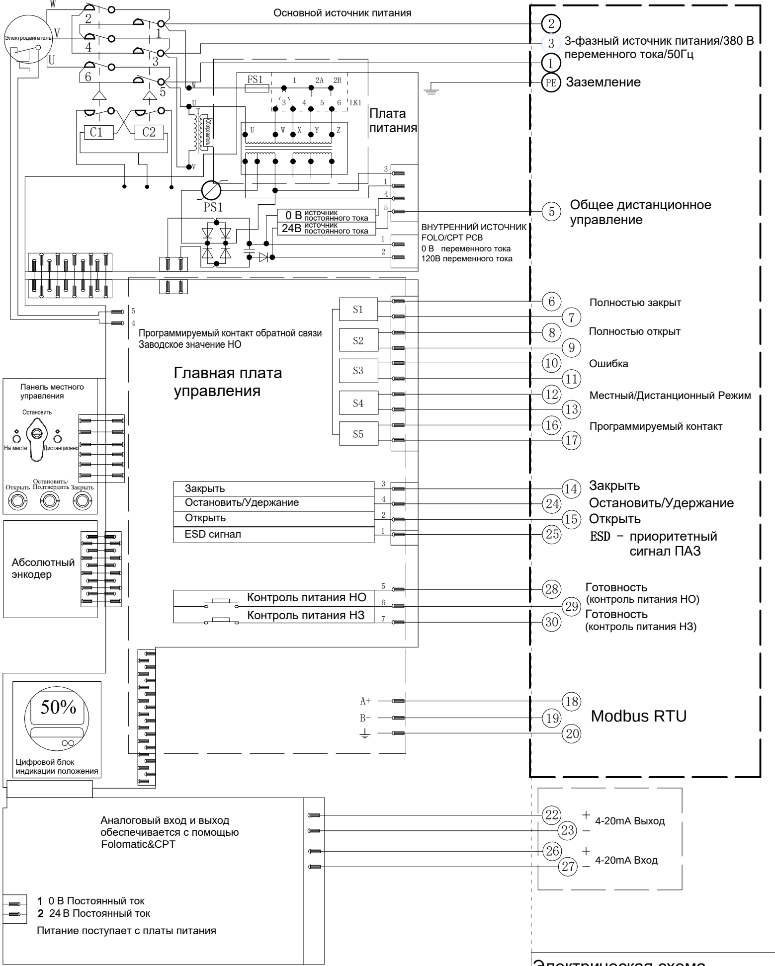
Электрическая схема №2-380-24-6-MR-1 Серия VADQ006-010-015-020-030/ VADQ100-150-200
