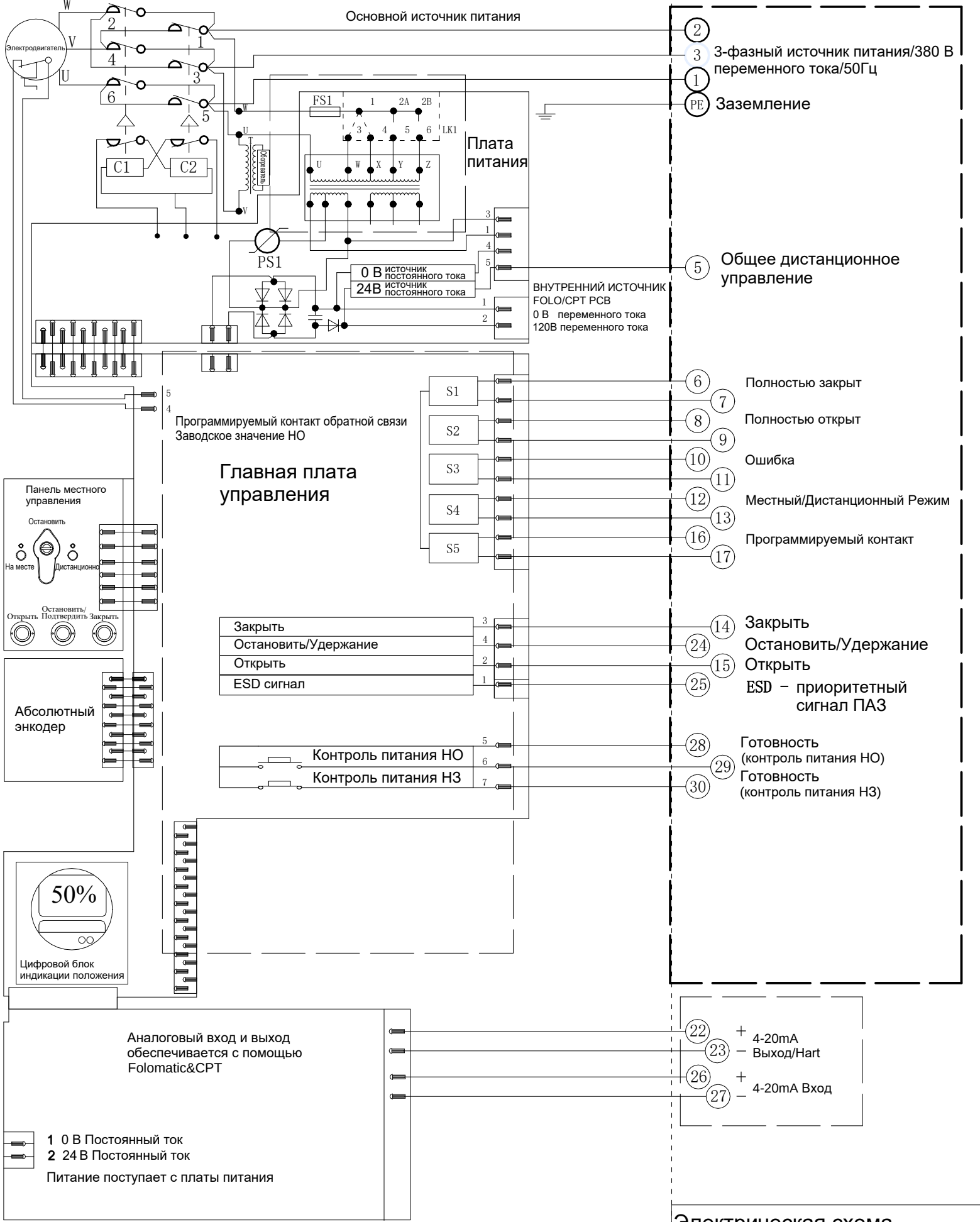
Электрическая схема №2-380-24-6-HR-1 Серия VADQ006-010-015-020-030/ VADQ100-150-200
