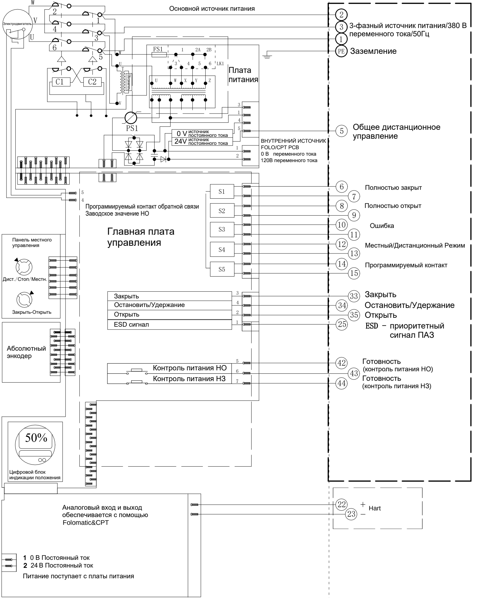
Электрическая схема № 3-380-24-6-HR-0
