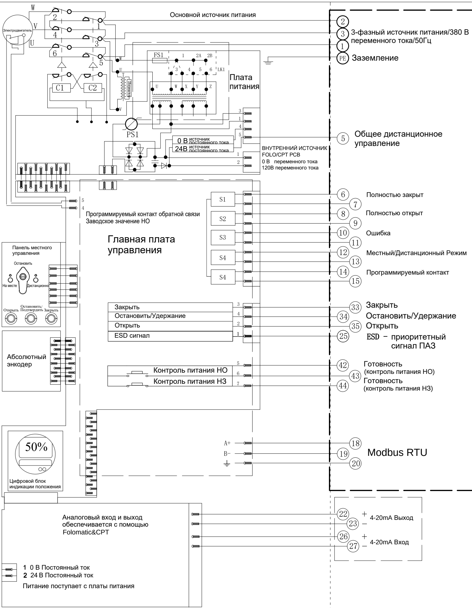
Электрическая схема №3-380-24-6-MR-1 Серия VADQ040/060/080
