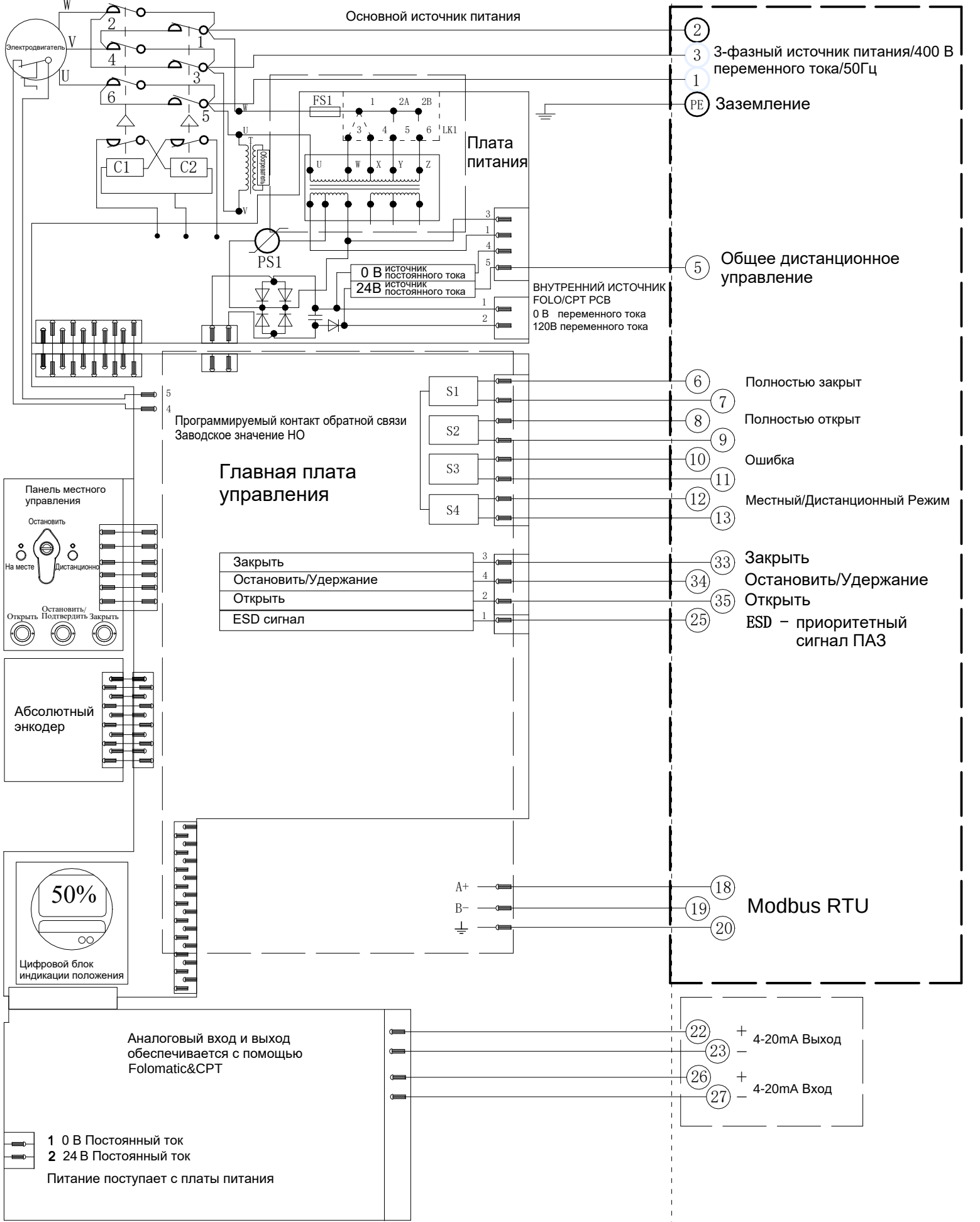
Электрическая схема №3-400-24-4-MR-1 Серия VADQ040/060/080
