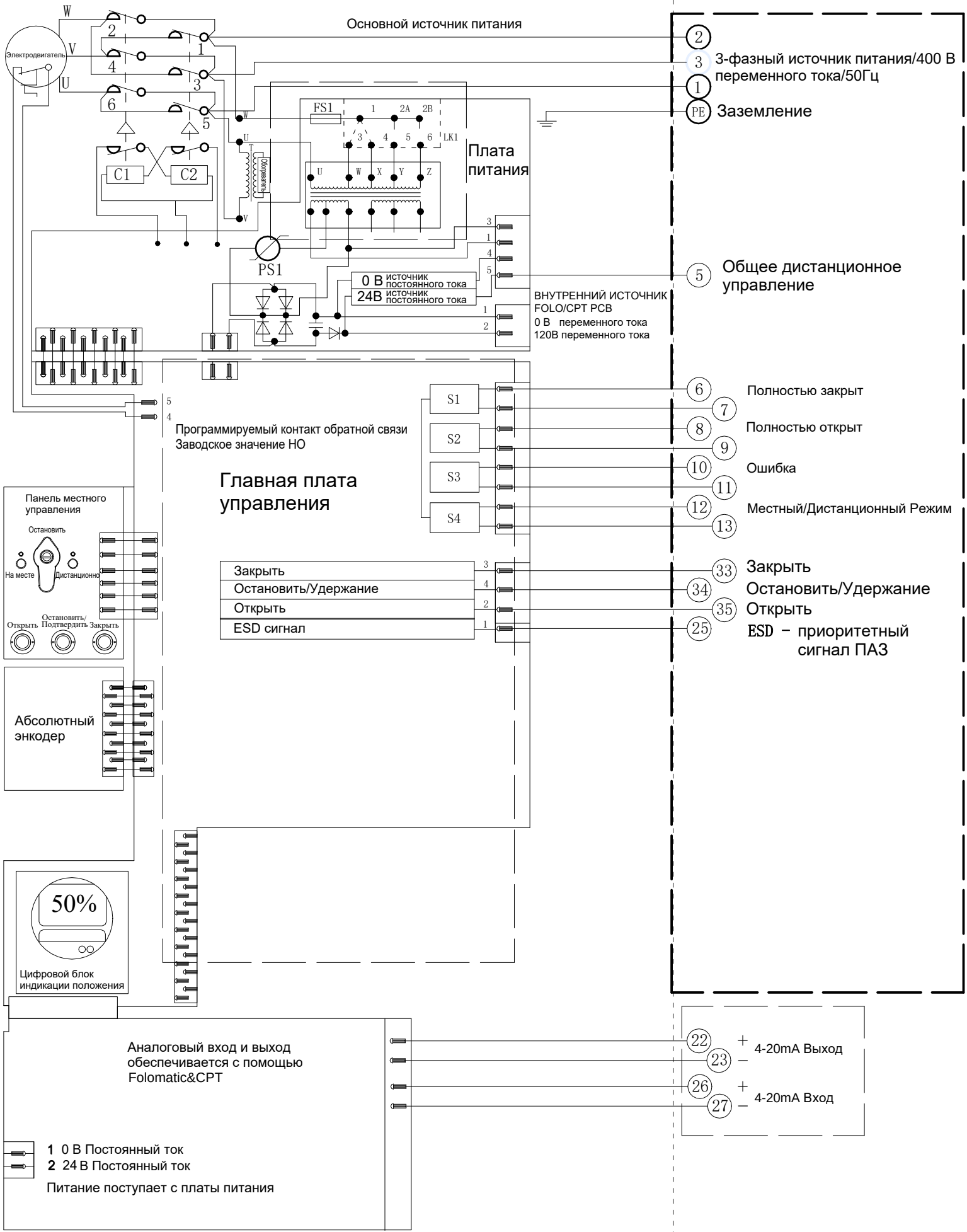
Электрическая схема №3-400-24-4-N-1 Серия VADQ040/060/080
