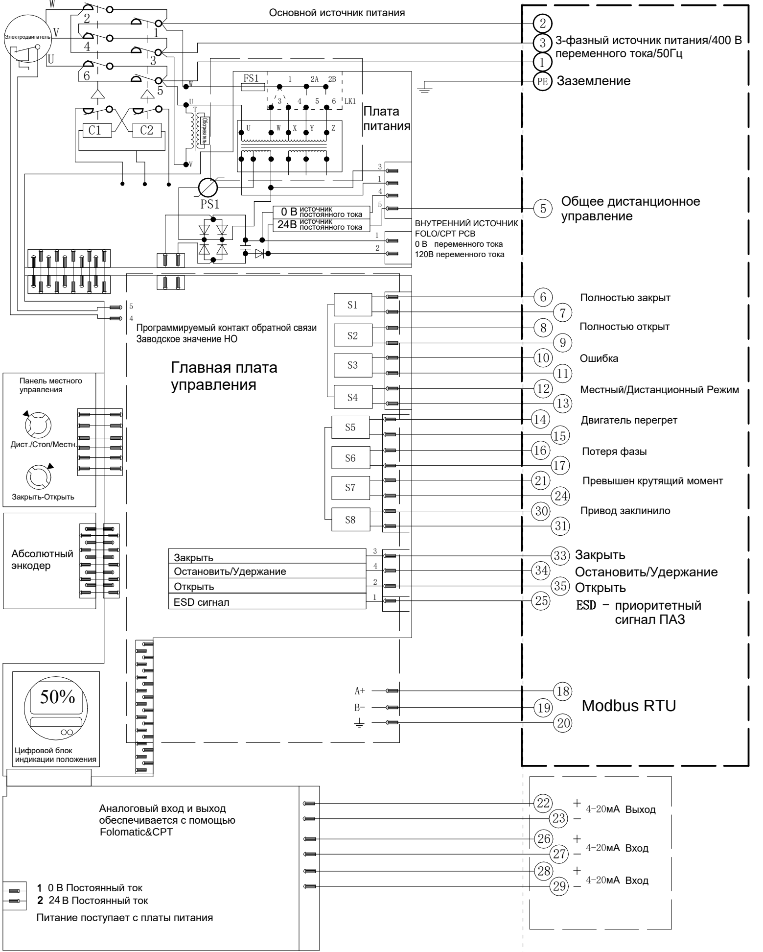
Электрическая схема № 3-400-24-8-MR-4 Серия VADQ040/060/080
