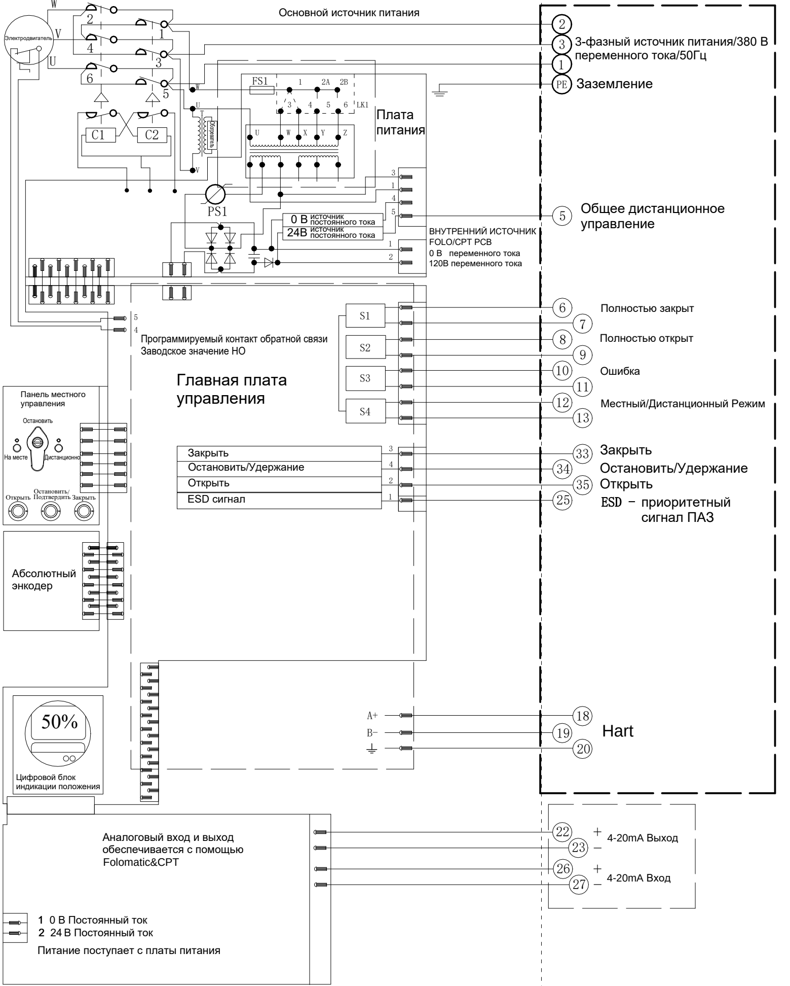
Электрическая схема №3-380-24-4-HR-1 Серия VADQ040/060/080
