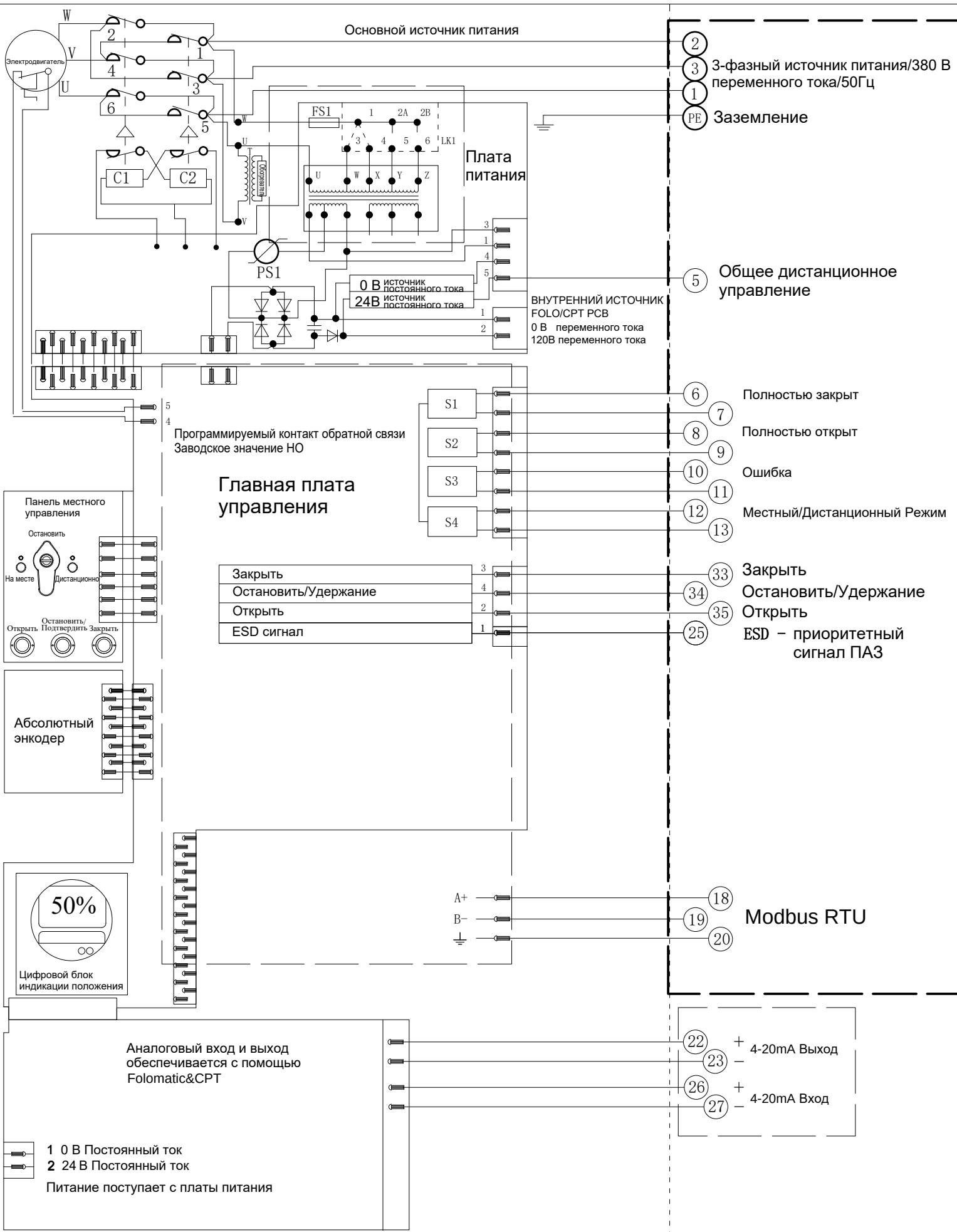
Электрическая схема №3-380-24-4-MR-1 Серия VADQ040/060/080
