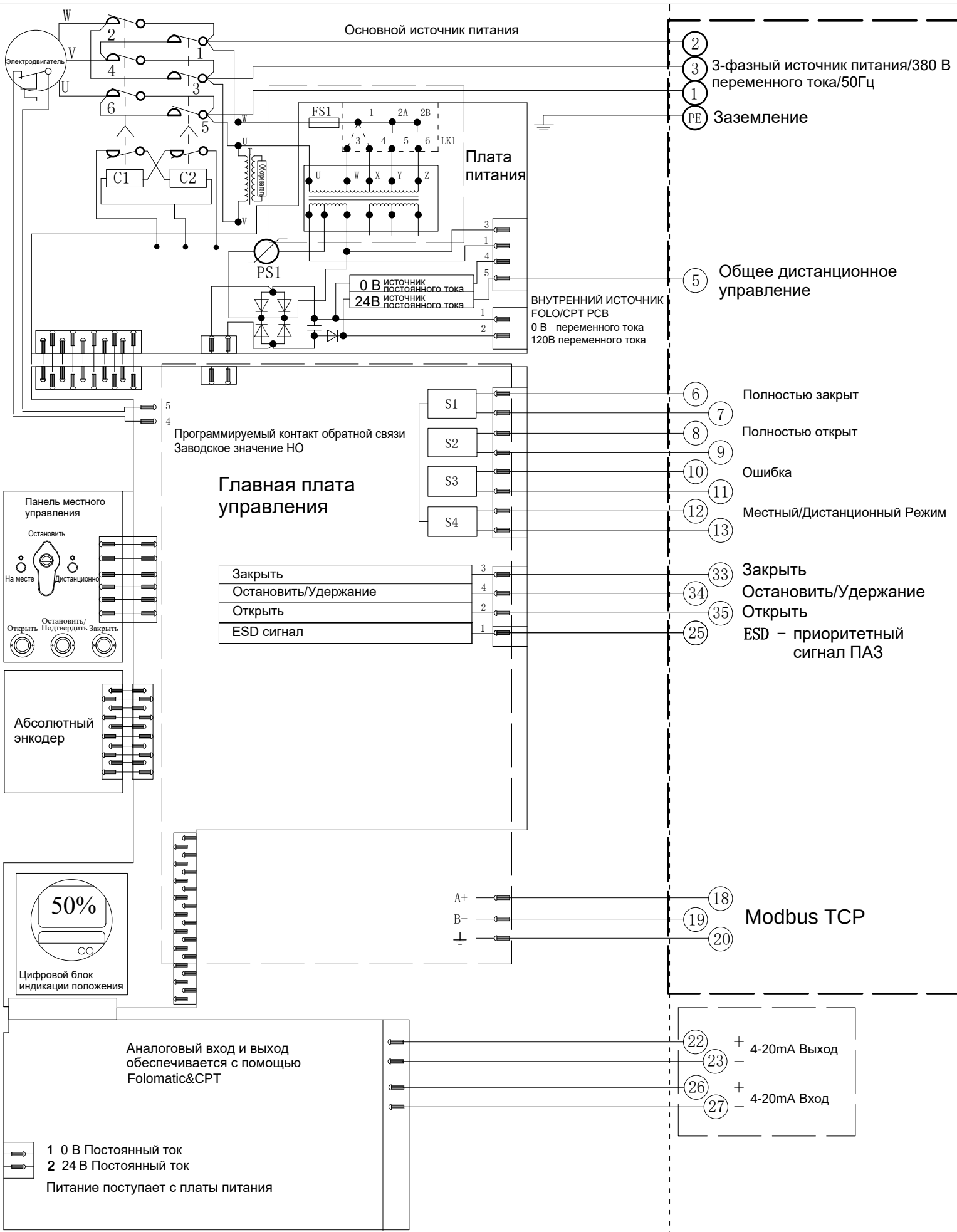
Электрическая схема №3-380-24-4-MT-1 Серия VADQ040/060/080
