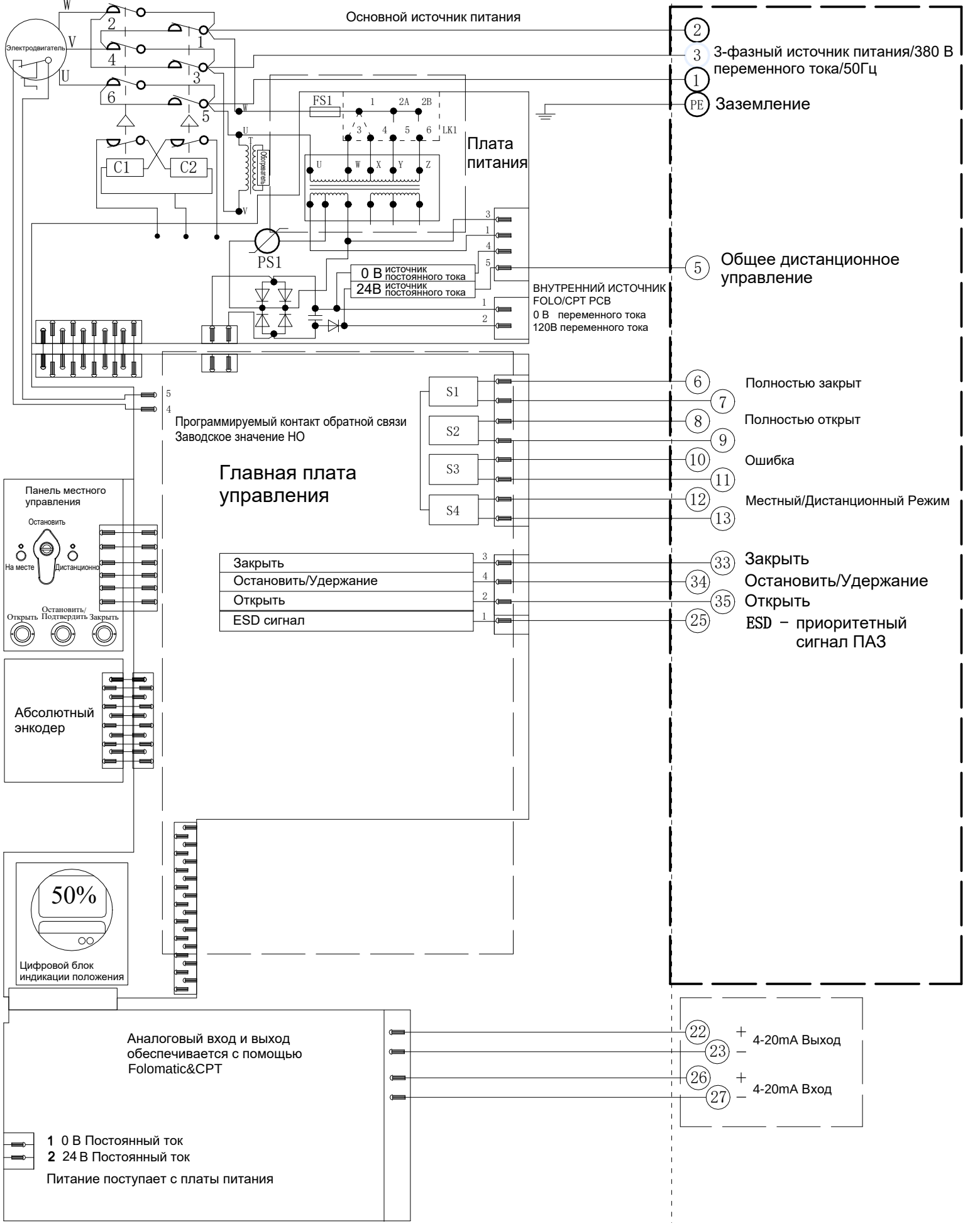
Электрическая схема №3-380-24-4-N-1 Серия VADQ040/060/080
