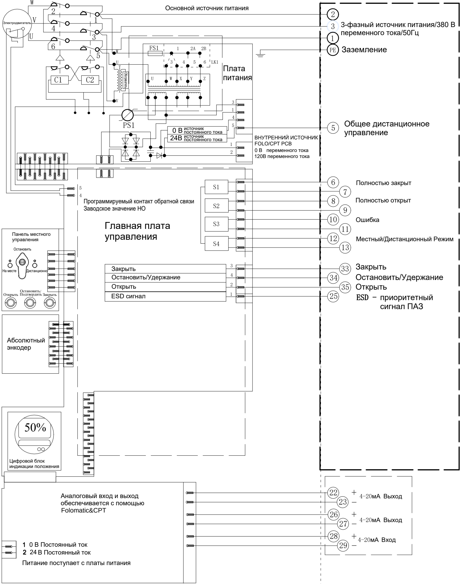
Электрическая схема №3-380-24-4-N-5 Серия VADQ040/060/080
