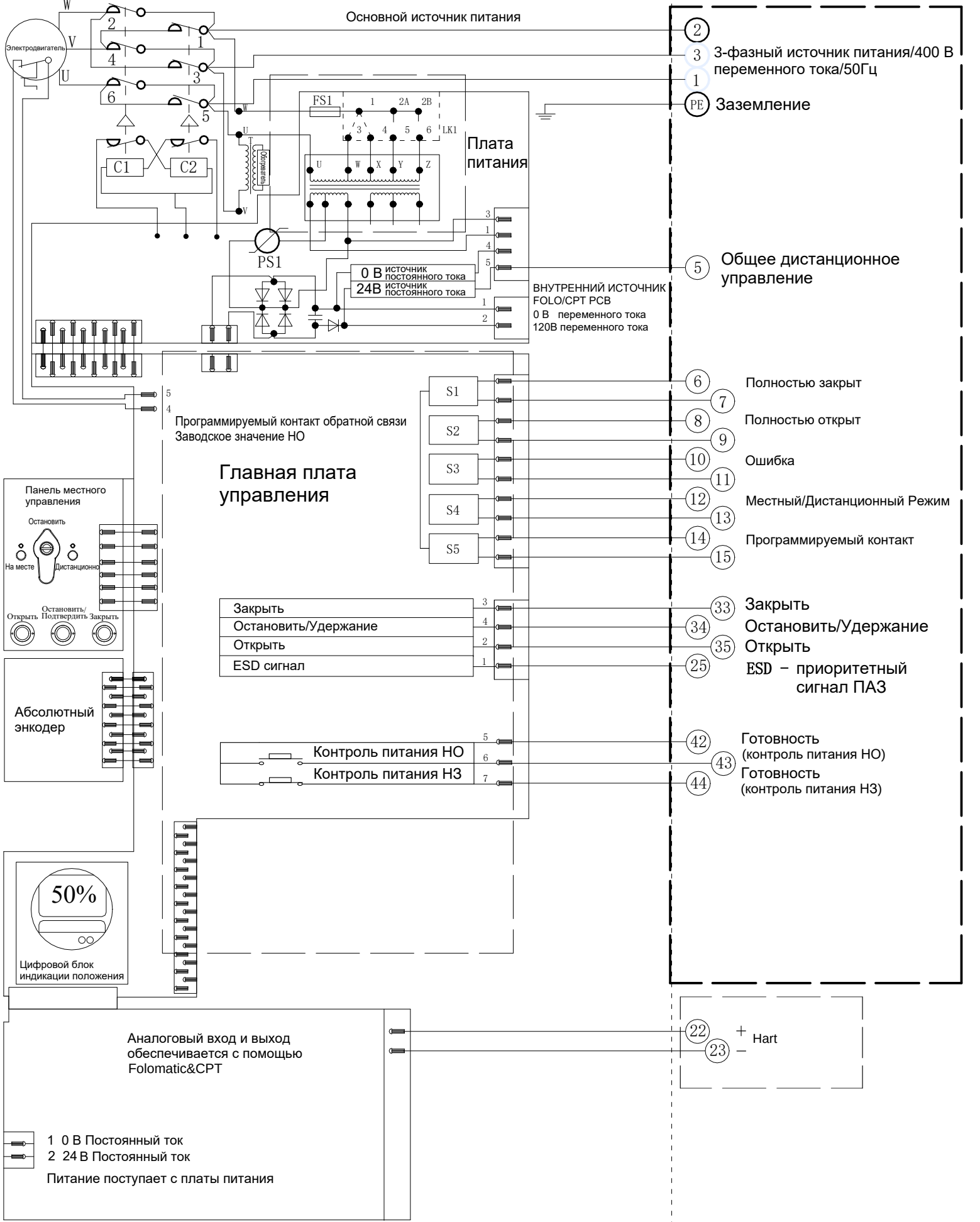
Электрическая схема №6-400-24-6-HR-0 Серия VADM
