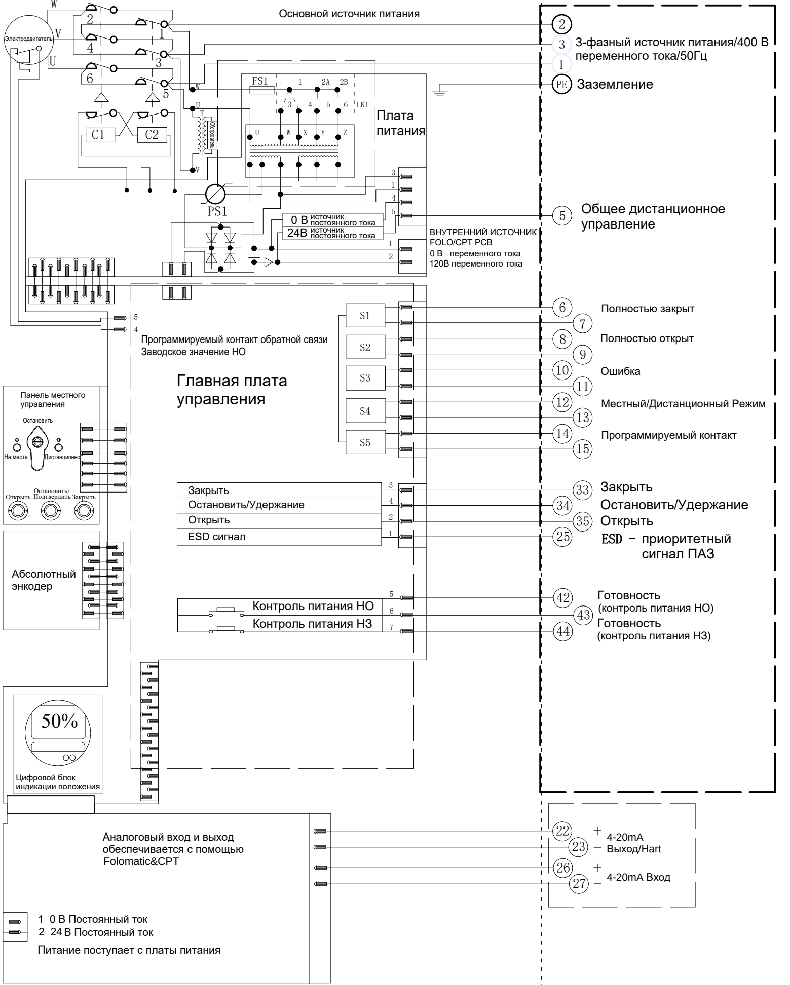
Электрическая схема №6-400-24-6-HR-1 Серия VADM
