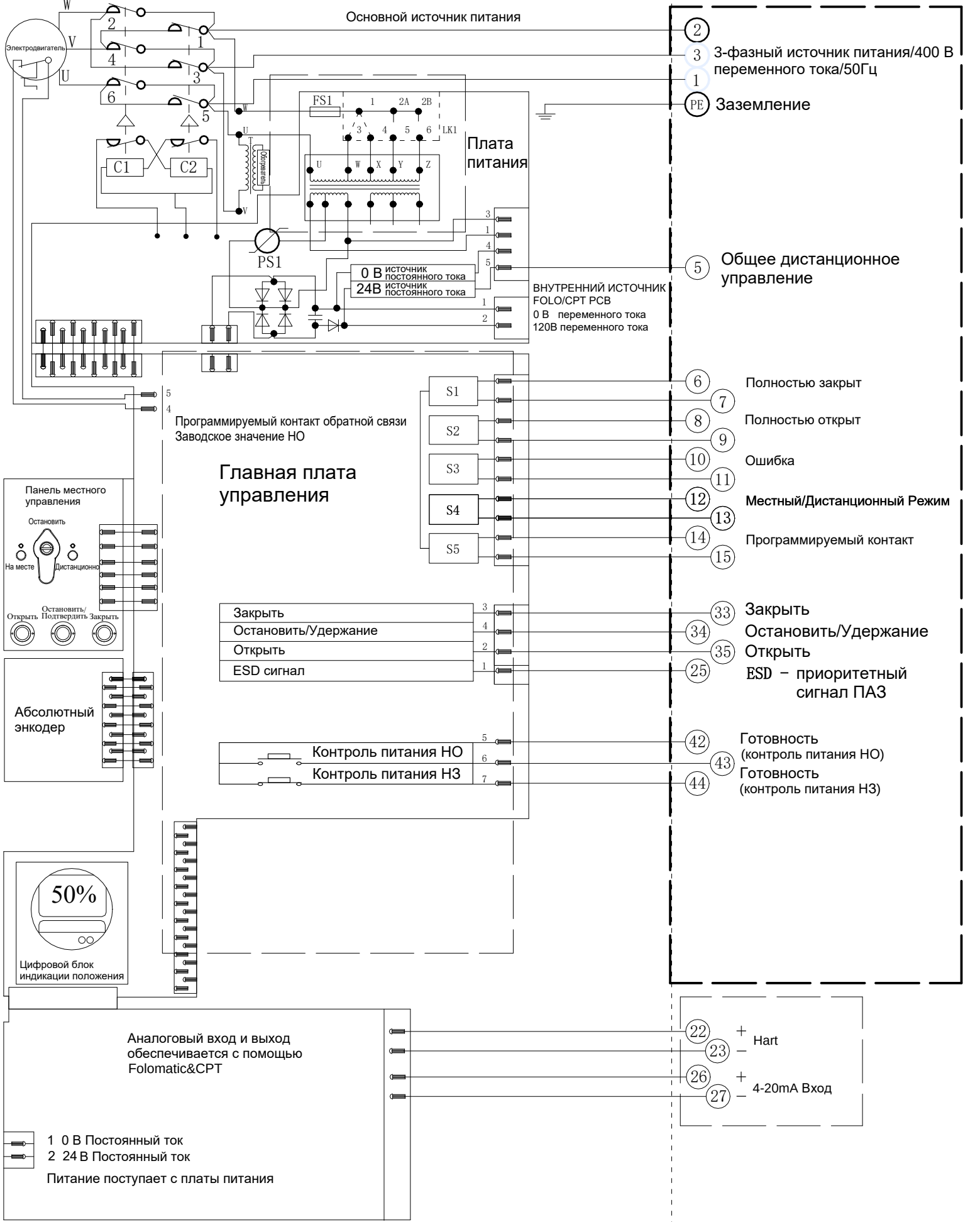
Электрическая схема №6-400-24-6-HR-2 Серия VADM
