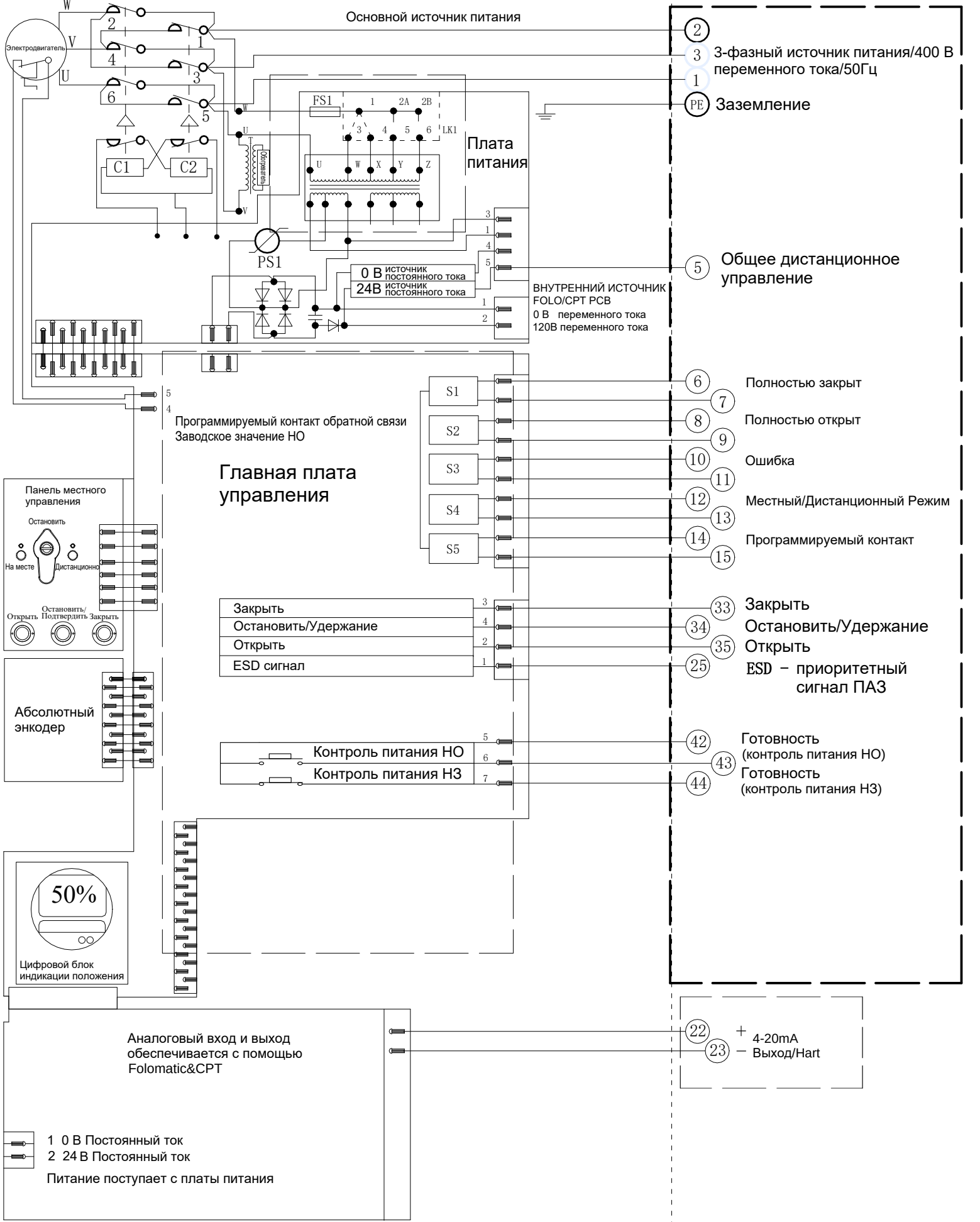
Электрическая схема №6-400-24-6-HR-3 Серия VADM
