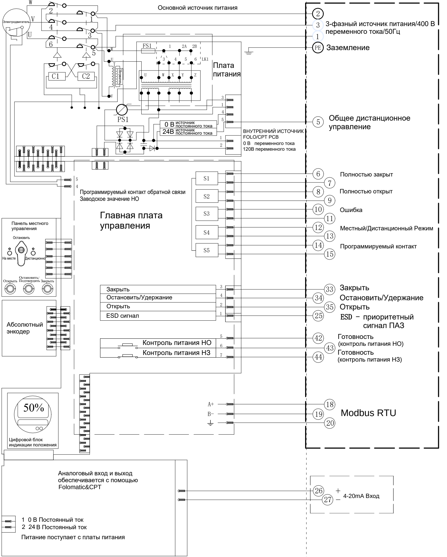
Электрическая схема №6-400-24-6-MR-2 Серия VADM
