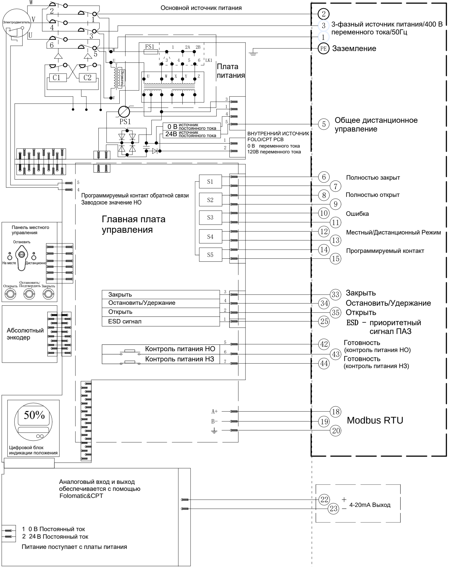
Электрическая схема №6-400-24-6-MR-3 Серия VADM
