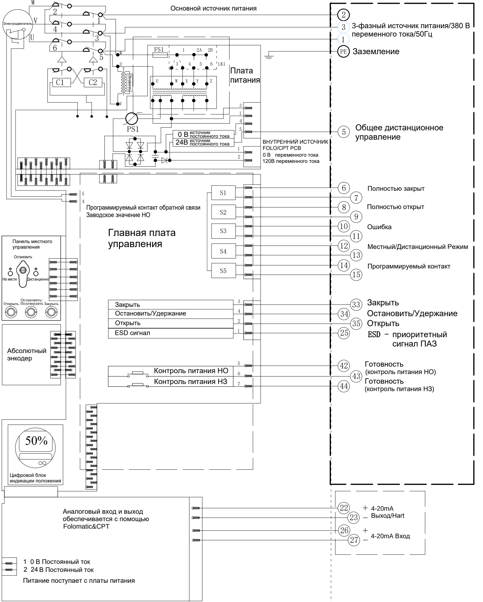
Электрическая схема №6-380-24-6-HR-1 Серия VADM
