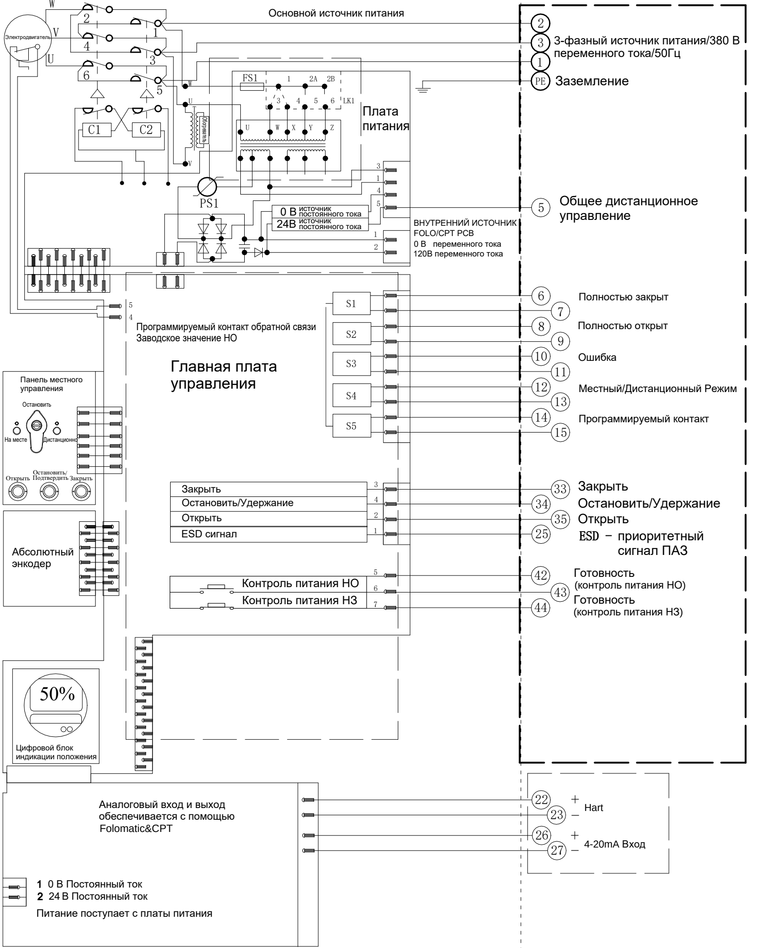
Электрическая схема №6-380-24-6-HR-2 Серия VADM
