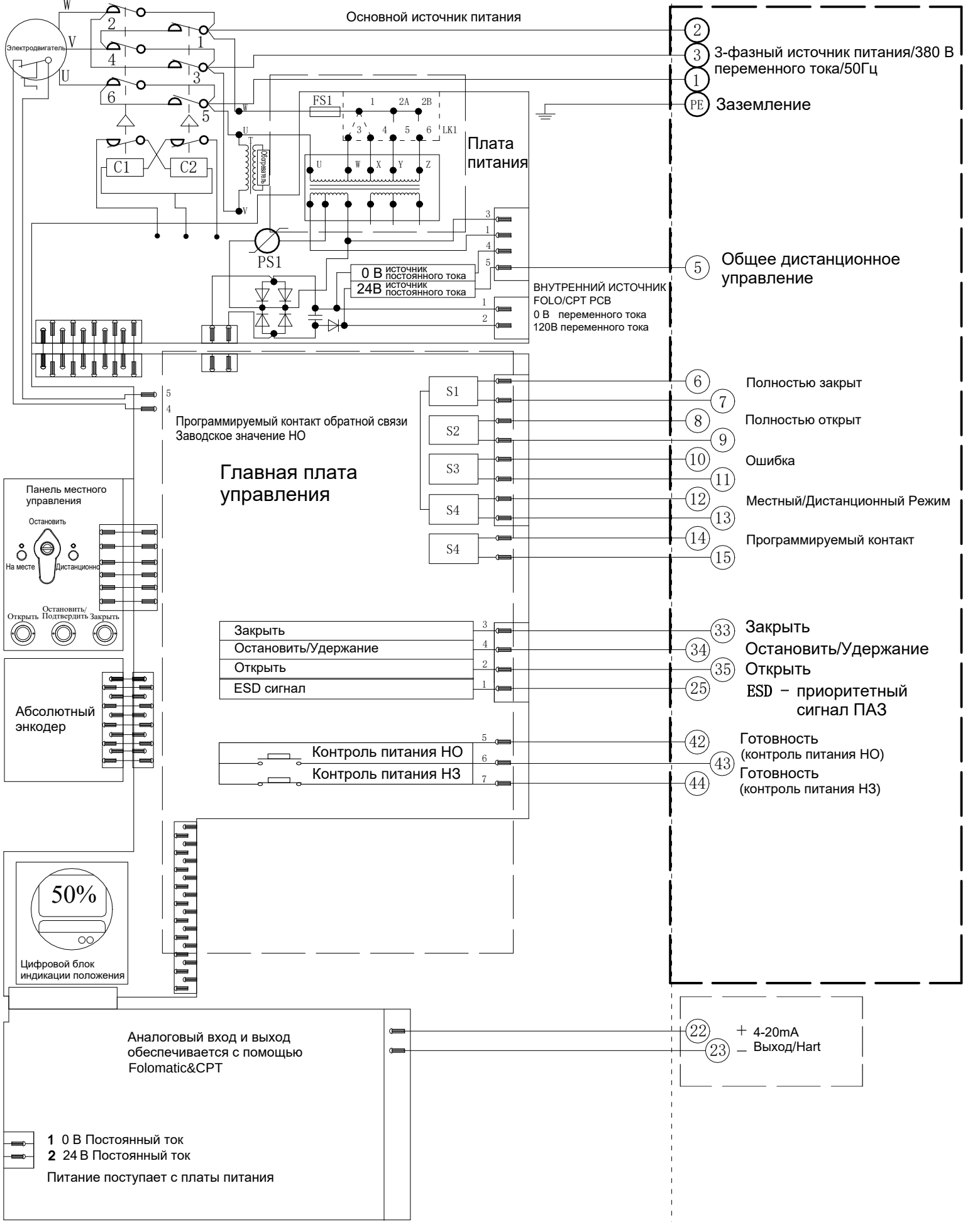
Электрическая схема №6-380-24-6-HR-3 Серия VADM
