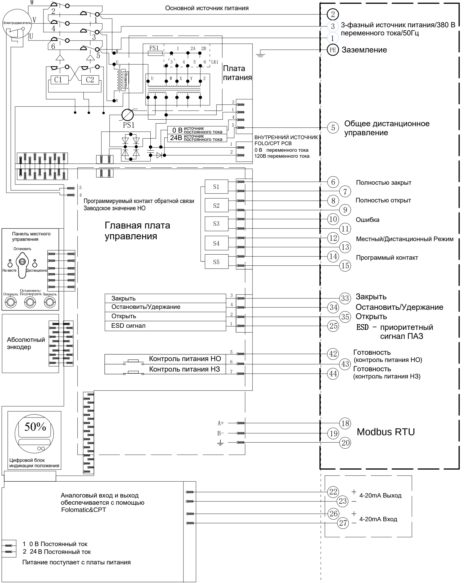
Электрическая схема №6-380-24-6-MR-1 Серия VADM
