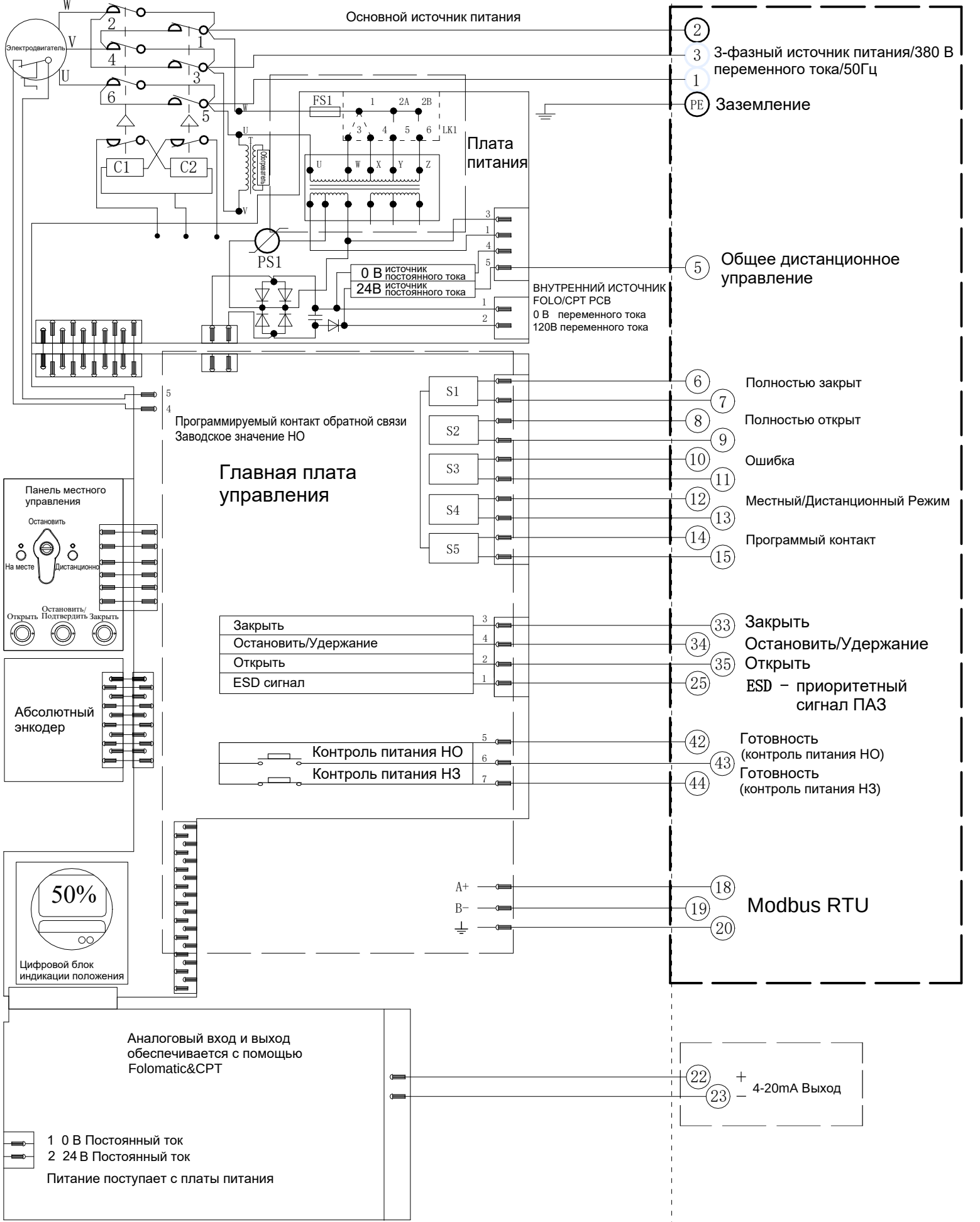
Электрическая схема №6-380-24-6-MR-3 Серия VADM
