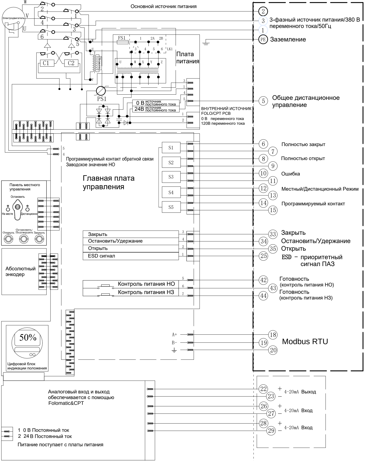
Электрическая схема №6-380-24-6-MR-4 Серия VADM
